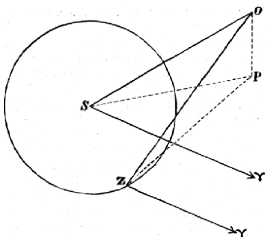
Č. 1675. Heliocentrická délka a šířka.
