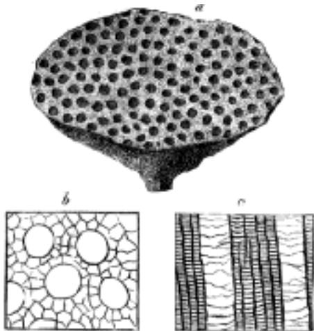
Č. 1676. Helioolithes megastoma z e 2 .
