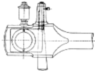
Č. 1711. Hlava ojníční.
