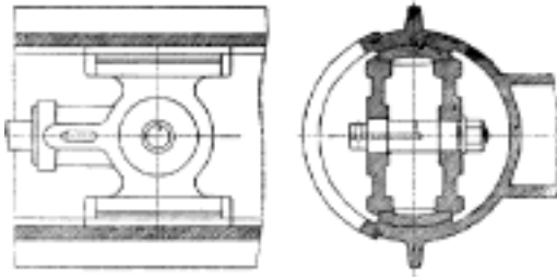
Č. 1710. Hlava křížová.
