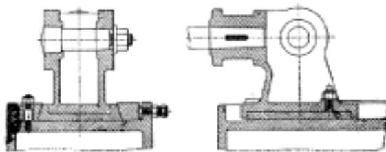
Č. 1709. Hlava křížová.
