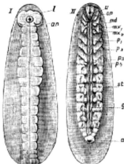
Č. 1724. Dvě stadia vývoje vodmily.
