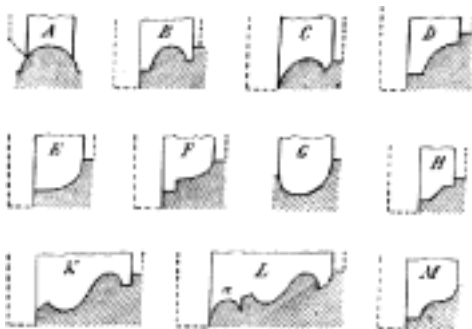
Č. 1728. Hoblíky truhlářské.
