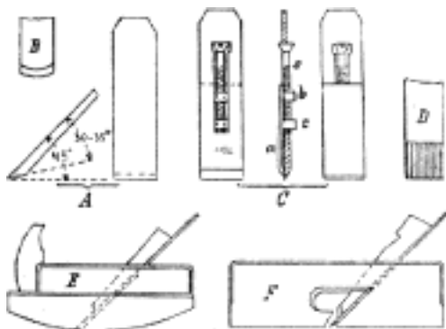
Č. 1726. Hoblíky truhlářské.
