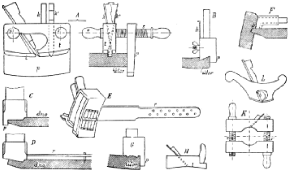
Č. 1729. Hoblíky bednářské a kotlářské.
