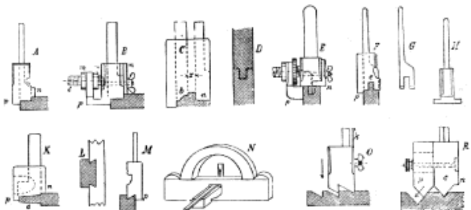
Č. 1727. Hoblíky truhlářské.
