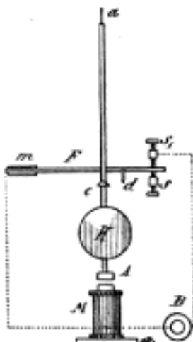
Č. 1738. Hippovy vlastní elektrické hodiny.
