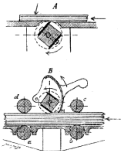
Č. 1732. Hoblovací stroj na dřevo (uspořádání nožů).
