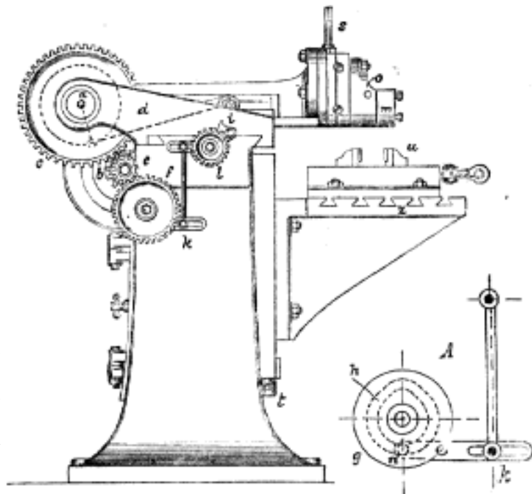
Č. 1730. Hoblovací stroj na kovy (shaping).
