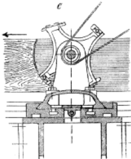
Č. 1732. Hoblovací stroj na dřevo (uspořádání nožů).
