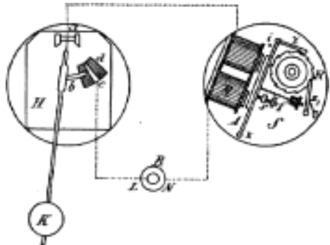
Č. 1736. Bainovy sympathetické, elektrické hodiny.
