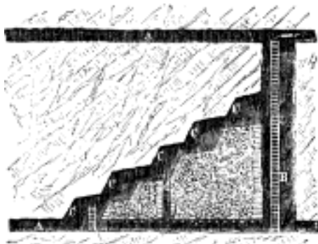
Č. 1763. Dobývání výstupkové.
