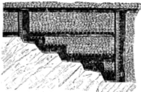
Č. 1762. Dobývání sestupkové.
