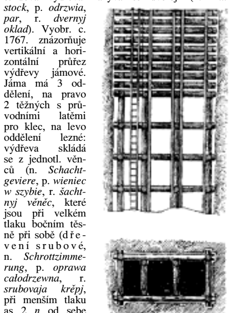
Č. 1767. Vertikální a horizontální průřez výdřevy jámové.
