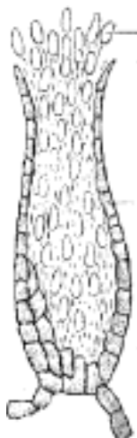
Č. 1787. Plodnice konidiová, o obal, k konidie.
