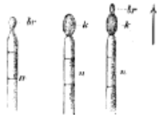
Č. 1785. Vytváření konidií. n nosič, br bradavka, k konidie.
