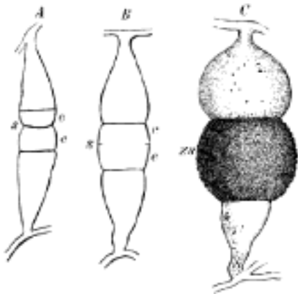
Č. 1788. Vytváření se zygosporu. A) Dvě vlákna myceliová při s odděli se přehrádkami cc. - B) Původní stěna se zrušila, obě buňky cc splynuly. - C) z mladá zygospora (90krát zvětšeno, Mucor stolonifer ).
