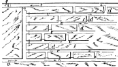
Č. 1771. Část větrné mapy.
