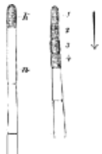
Č. 1786. Vytváření konidií. n nosič, k 1-4 konidie.
