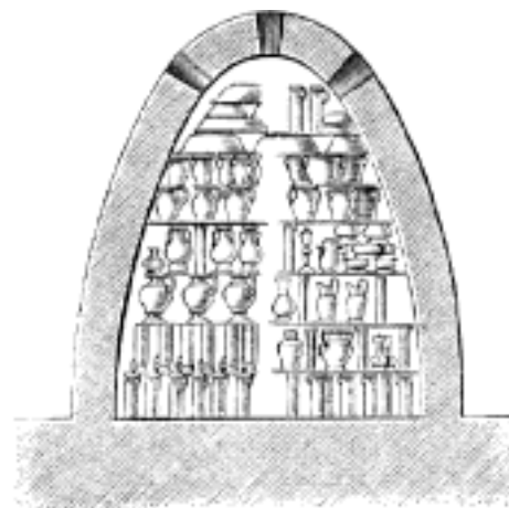
Č. 1812. Uložení zboží hrncířského v peci.
