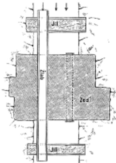
Č. 1805. Hráz přímá (v hornictví).
