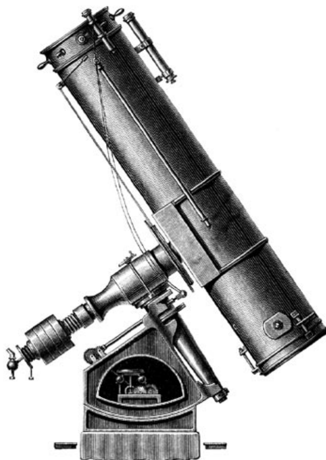
Čís. IV. Grubbův tvar reflektorů newtonských.
