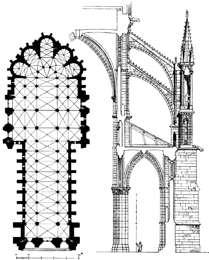
Kathedrála v Remeši (dle Viollet-le-Duca) Půdorys Opěrný systém
