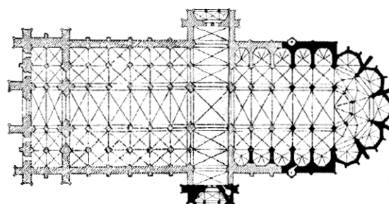
Původní půdorys chrámu sv. Víta od Matiaše z Arrasu
