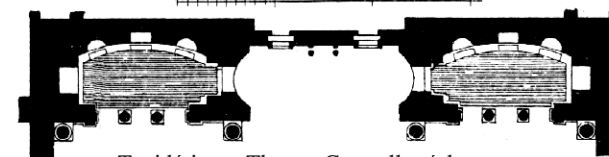
Tepidárium z Therem Caracallových Ideální řez dle Violet-le-Duca
