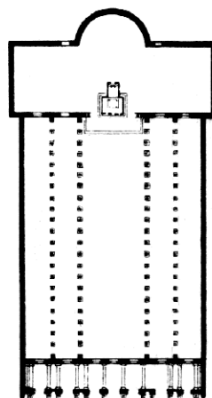
Půd. bas. sv. Pavla
