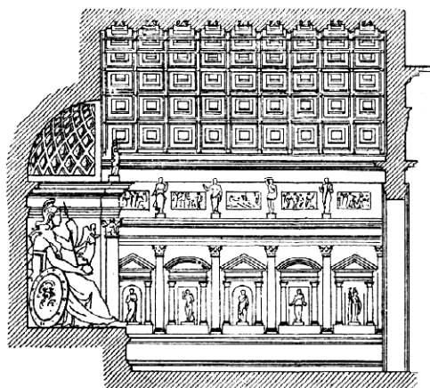
Podélný řez
