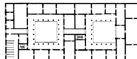
Řecký dům (dle Beckera)
