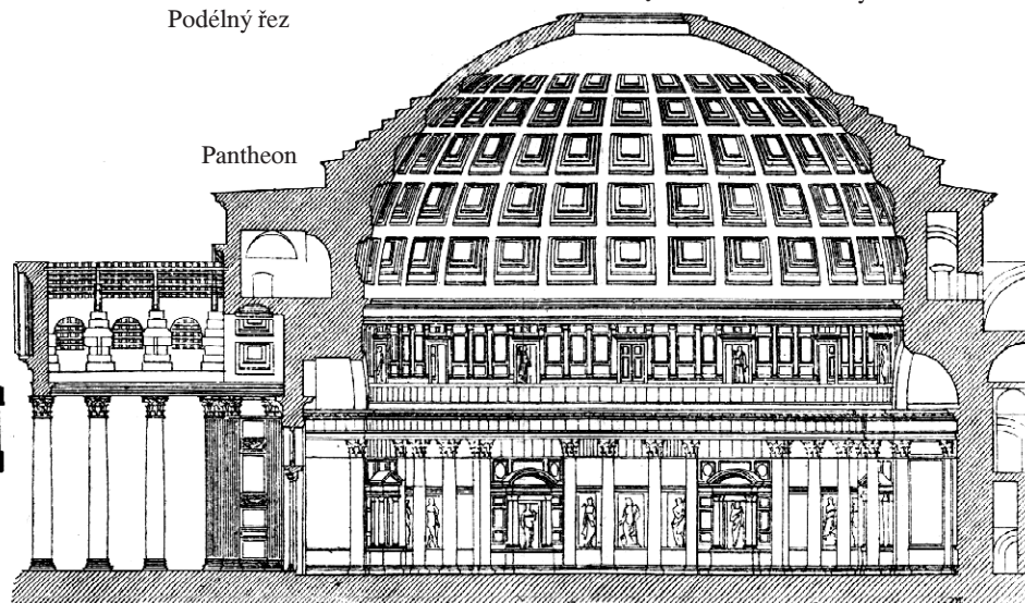
Podélný řez
