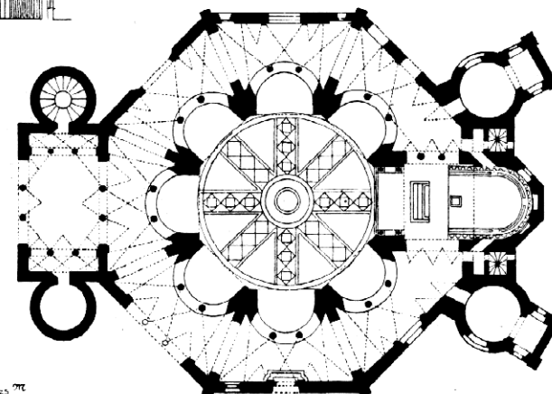
San Vitale v Ravenně řez a půdorys
