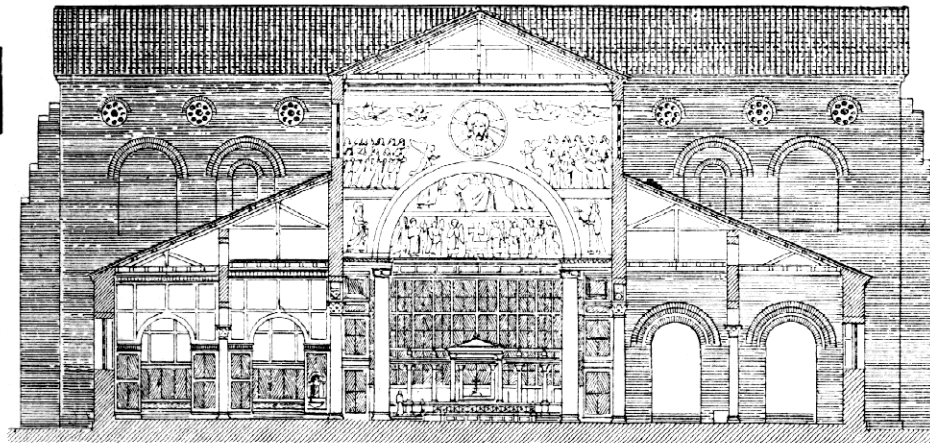
Řez bas. sv. Pavla
