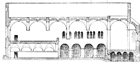
Podélný řez
