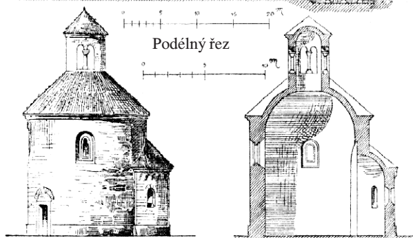
Kaple sv. Kříže v Praze
