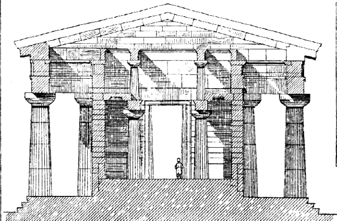
Rez chrámem Poseidona v Paestum
