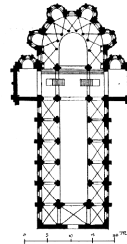
Notre Dame du Port půdorys
