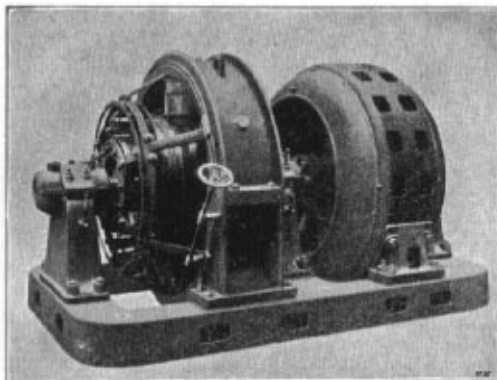
Rotační transformátor (Elektrot. akc. spol. dříve Kolben a spol., Vysočany).
