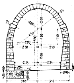
TUNNEL SIMPLONSKÝ
