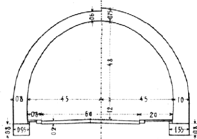
TUNNEL VYŠEHRADSKÝ
