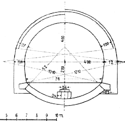
SV. GOTTHARD
