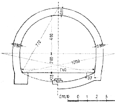
MONT-CENIS.
