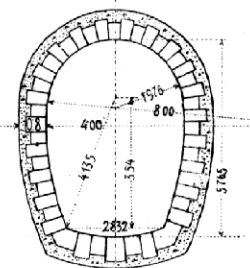
MONT-CENIS.
