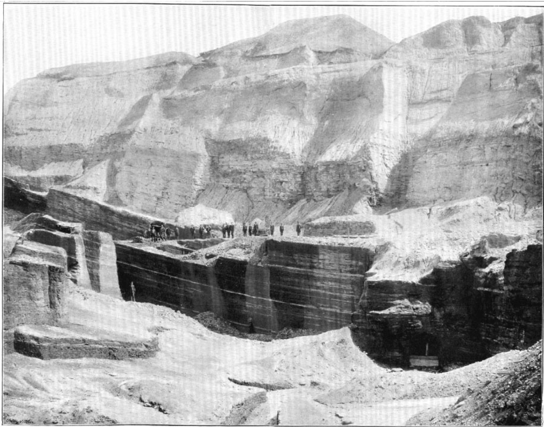
Výchoz svrchní radnické sloje kamenouhelné v odklizu hraběte Šternberka blíže Vranovic u Radnic.
