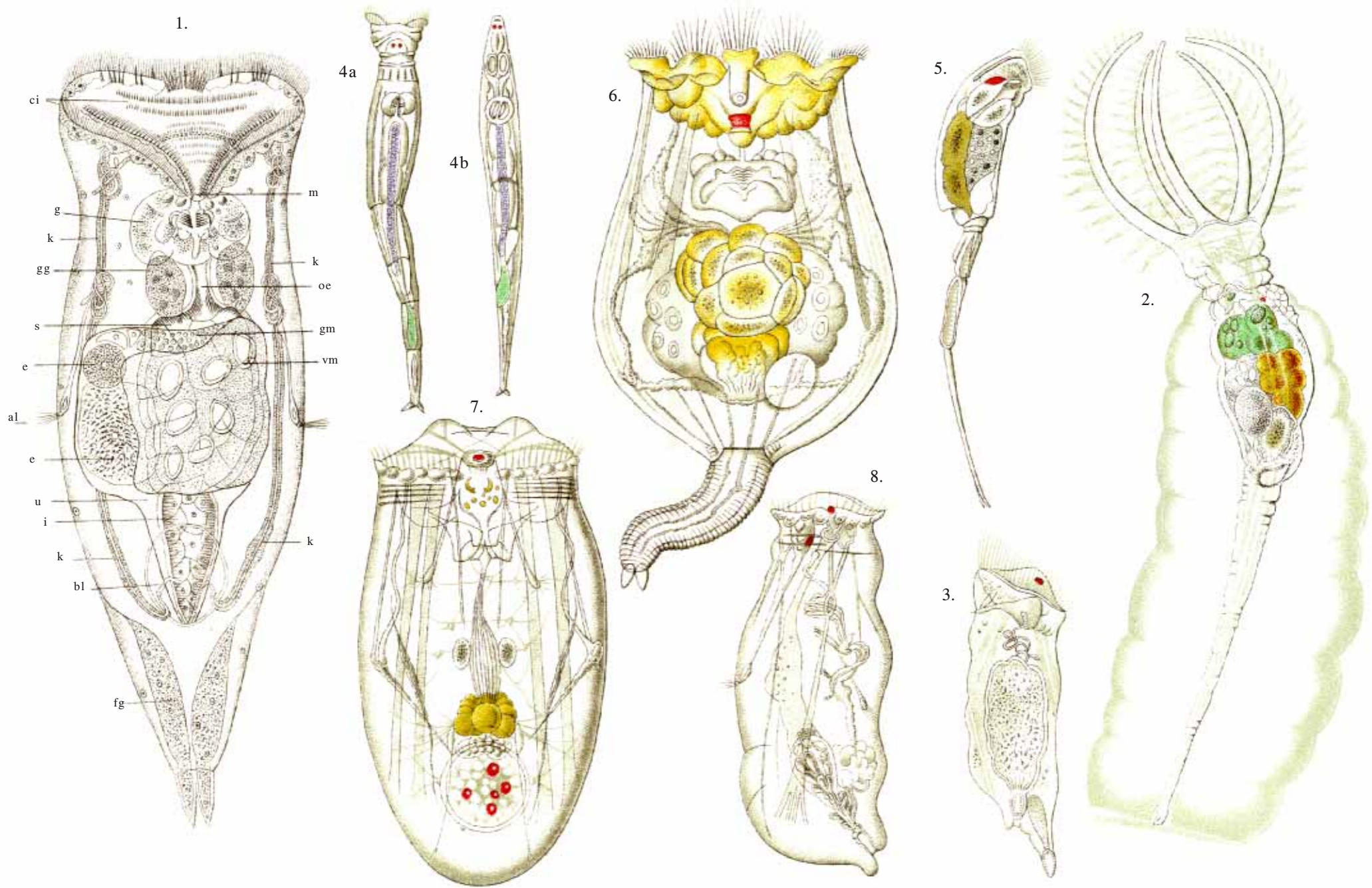
1. Hydatina senta Ehrbg. (ci ústroj vířivý, m ústa, g ústroj žvýkací, k soustava exkreční či vyměšovací, oe jícen, gg žlázy žaludeční, s žaludek, gm zárodečná část vaječníku, vm žloutková část vaječníku, e vajíčko, al postranní ústroj smyslový, u vejcovod, i konečník, bl ztažitelný váček, fg žláza nožní). - 2. Stephanoceros Eichhornii Ehrbg. - 3. Lacinularia socialis Ehrbg. (sameček). - 4a, 4b. Rotifer vulgaris Ehrbg. 5. Scaridium longicaudum Ehrbg. - 6. Brachionus urceolaris Ehrbg. - 7. Asplanchna priodonta Gosse (samička). - 8. Asplanchna priodonta Gosse (sameček). - Vše silně zvětšeno.
