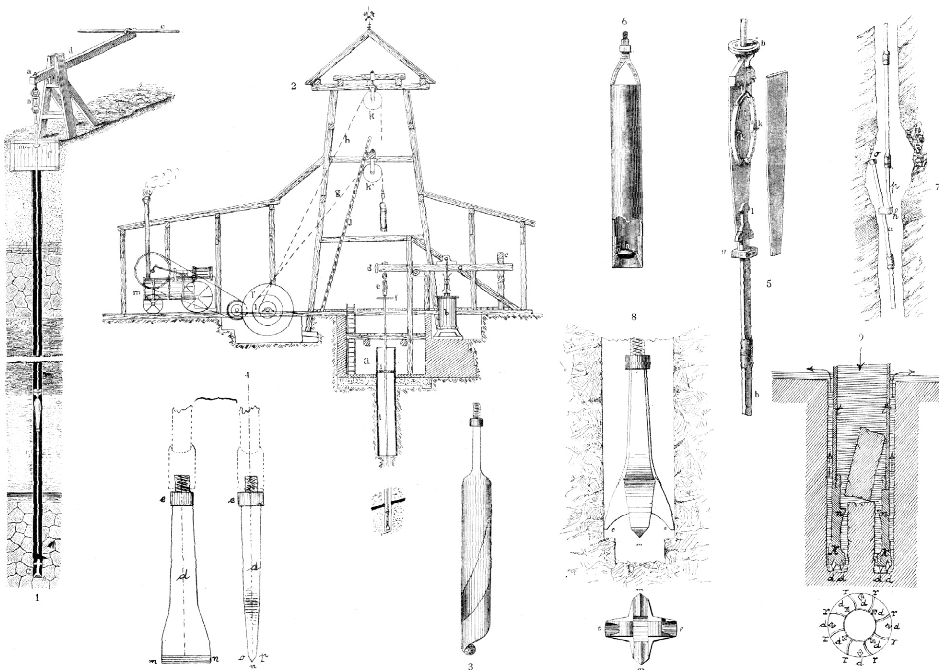
1. Ruční vrtání razivé. - 2. Vrtání parou. - 3. Zemní nebozez točivý. - 4. Dřátový nebozez. - 5. Kindův spadák. - 6. Lýžka čili šlamovka. - 7. Lapací pazour. - 8. Příběrák. - 9. Diamantový nebozez.
