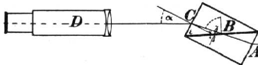
Č. 3454. Refraktometr Abbeův.
