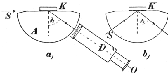
Č. 3455. Refraktometr Abbeův v novější úpravě.
