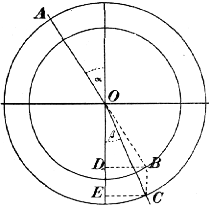
Č. 3458. Reuschova konstrukce paprsku lomeného.
