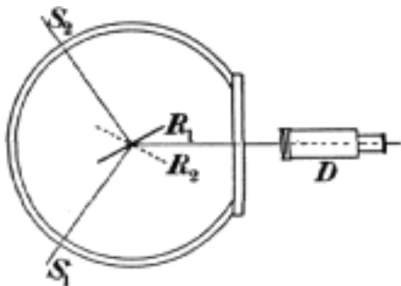
Č. 3453. Totální reflektometr Kohrauschův.
