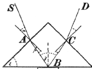
Č. 3452. Hranol Wollastonův.
