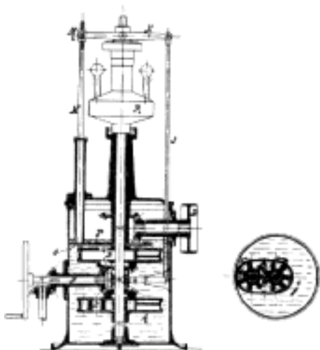
Č. 3471. Hydraul. regulátor firmy Escher, Wyss a spol.
