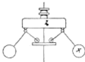
Č. 3469. Regulátor cosinusový.
