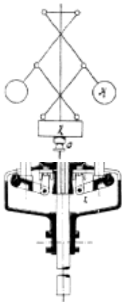
Č. 3464. Regulátor Beyerův. Č. 3465. Hydraulický regulátor firmy Escher a Wyss. Č. 3466. Regulátor Kleyův.
