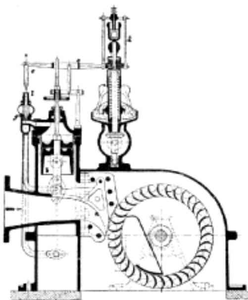
Č. 3464. Regulátor Beyerův. Č. 3465. Hydraulický regulátor firmy Escher a Wyss. Č. 3466. Regulátor Kleyův.
