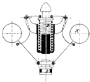
Č. 3463. Regulátor Pröllův.
