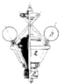
Č. 3467. Regulátor Hartungův.
