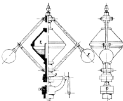
Č. 3461. Regulátor působící na škrtkci klapku. Č. 3462. Regulátor Porterův.
