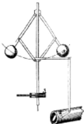
Č. 3461. Regulátor působící na škrtkci klapku. Č. 3462. Regulátor Porterův.
