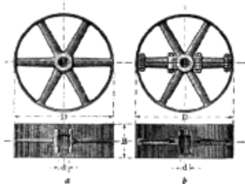
Č. 3487. a Řemenový kotouč litinový jednotný. b Řem. kotouč litinový dvoudílný.
