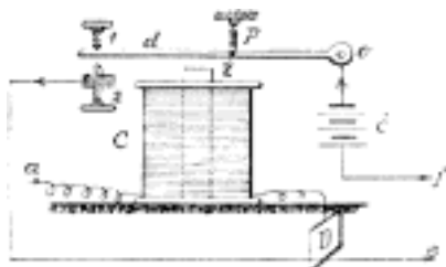
Č. 3477. Relais (princip).
