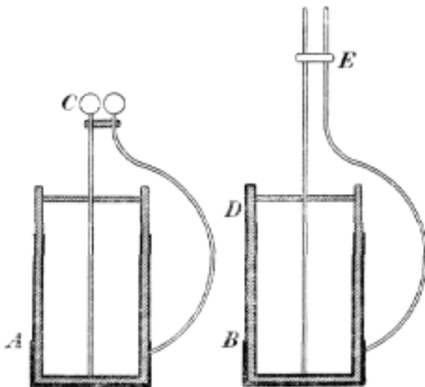
Č. 3495. Resonance elektrická: Pokus Lodgeův.
