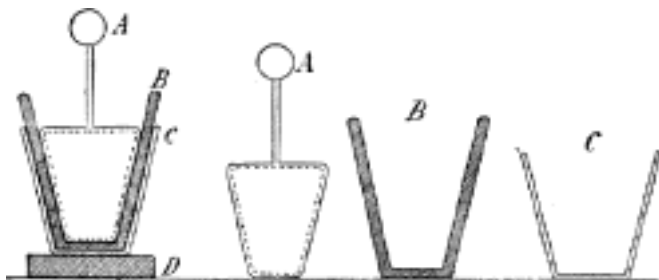
Č. 3494. Rozkladná láhev lejdská.
