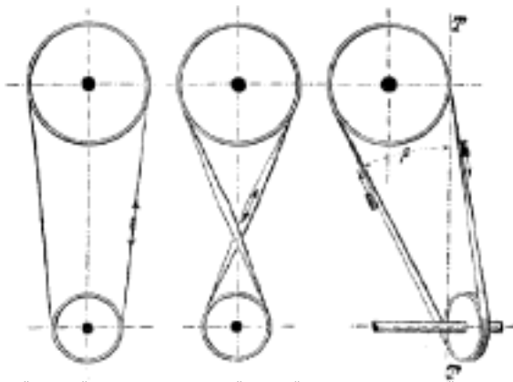
Č. 3482. Řem. opásání otevřené. Č. 3483. Řem. opásání zkřížené. Č. 3484. Řem. opásání polozkřížené.
