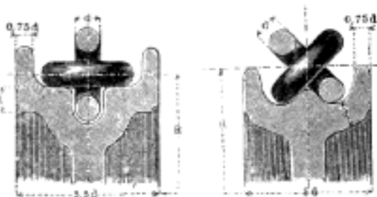
Č. 3499. Způsoby vedení řetězu na kotoučích.
