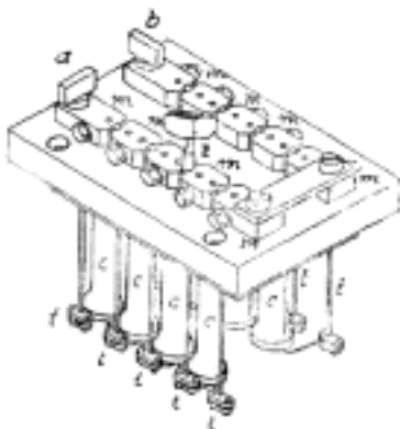
Č. 3513. Zátkový rheostat.
