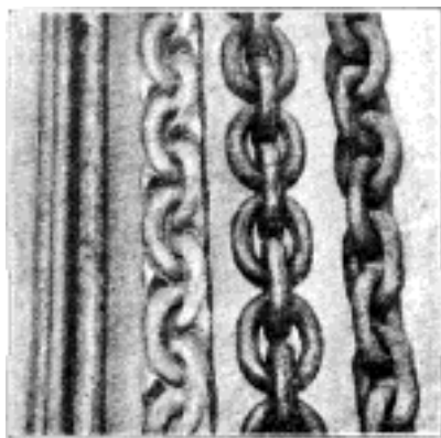
Č. 3505. Postup výroby řetězů válcováním.
