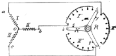
Č. 3519. Rheostat třífázový (spojení hvězdkové).
