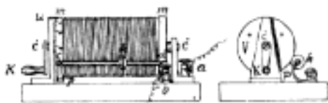
Č. 3512. Rheostat Wheatstoneův.
