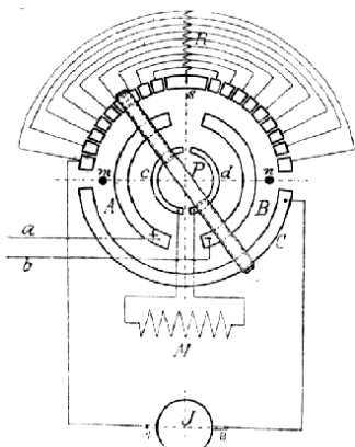
Č. 3518. Reversní rheostat.
