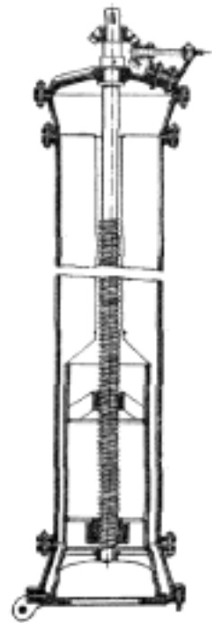
Č. 3562. Stroj na formování rour.
