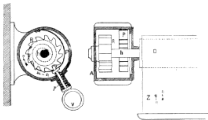
Č. 3556. Rouleau pérové.
