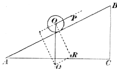
Č. 3576. Rovina nakloněná.
