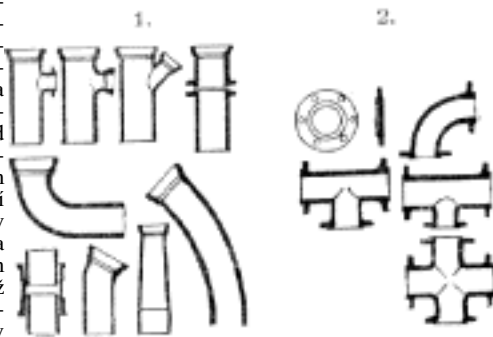
1. 2. Č. 3560. Kusy faconové 1. pro roury hrdlové. 2. pro roury flanšové.
