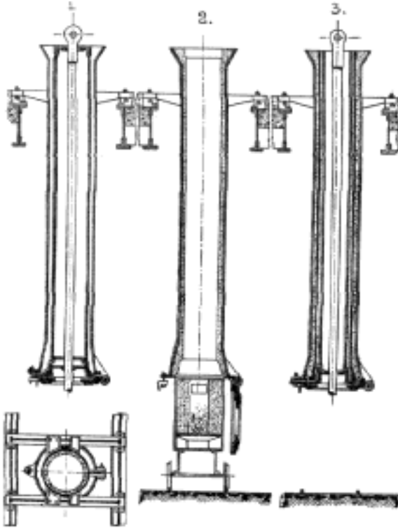
Č. 3561. 1. Forma pro rouru hrdlovou. 2. Vysušení formy. 3. Forma připravená k lití.
