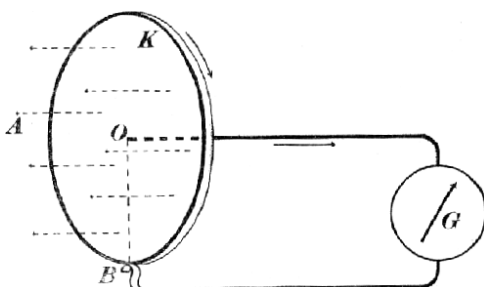
Č. 3551. Rotační induktor.
