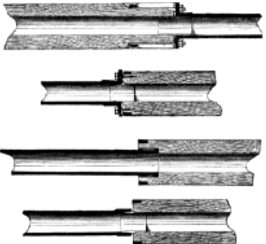
Č. 3569. Spojení rour dřevěných se železnými.
