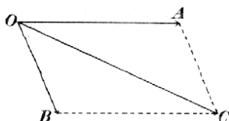
Č. 3579. Rovnoběžník sil.
