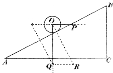
Č. 3575. Rovina nakloněná.
