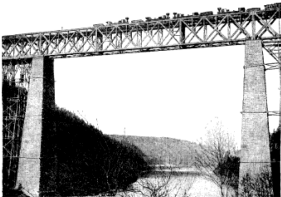
Č. 965. Viadukt nad Vltavou u Červené při zkoušce obtěžování.
