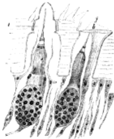
Č. 972. Průřez tykadlem vosy se 2 čichacími tyčinkami t, j jamka čichová s blankou b.
