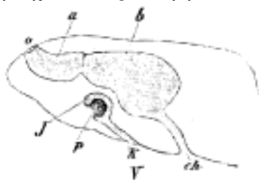
Č. 974. Schematický průřez lebky ještěrky. o zevní otvor čichový, ch zadní otvor č. choana, a přední, b zadní dutina nosní, j Jakobsonův orgán na papile p, k kanálek jeho a otvor do úst.
