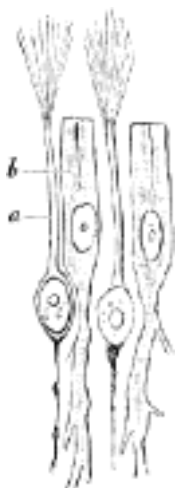
Č. 973. Čichová sliznice mloka. a buňky čichové, b buňky epithelové.
