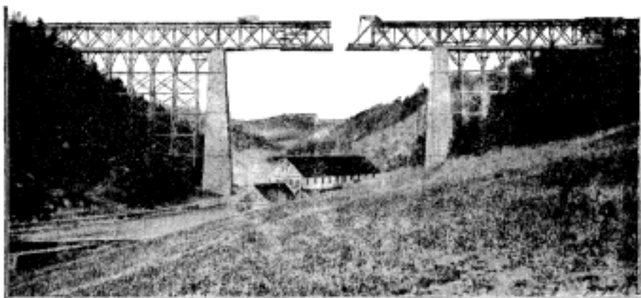
Č. 964. Viadukt nad Vltavou se středním polem nehotovým.
