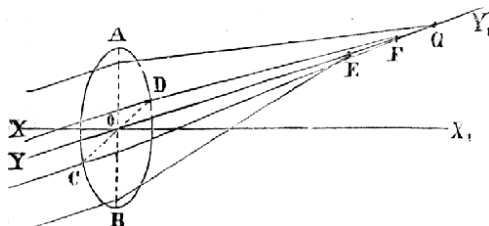
Č. 1014. Astigmatismus šikmých paprsků.
