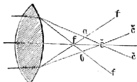
Č. 1012. Vada barevná u spojky.
