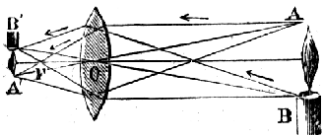
Č. 1008. Skutečné obrazy spojky.
