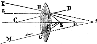
Č. 1007. Geometrický obraz bodu u spojky.
