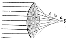
Č. 1013. Vada kulová (sferická).
