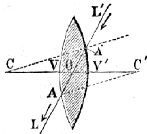
Č. 1003. Optický střed.
