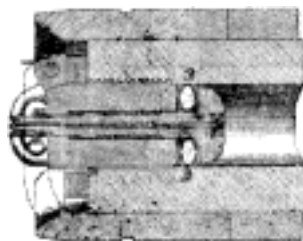
Č. 1094. Závor šroubem u francouzského děla polního. BB Ucpávka Bangeova.
