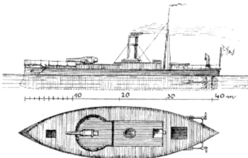
Č. 1106. Dělová lodice německá »Wespe«.
