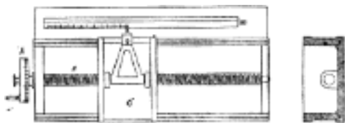
Č. 1080. Dělicí stroj přímý.
