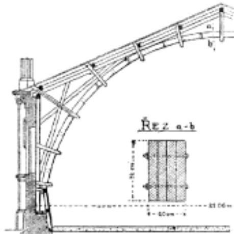
Č. 1104. Delormovy zkrúže ve vojenské jízdně pořícké v Praze.
