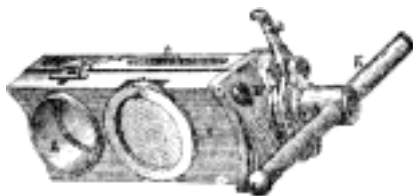
Č. 1097. Rakouský klin závor ní, pohled ze zadu.
