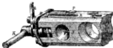
Č. 1098. Rakouský klin závor ní, pohled zepředu.
