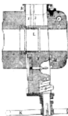
Č. 1096. Rakouský závor klinem; otevřený (průřez vodorovný).
