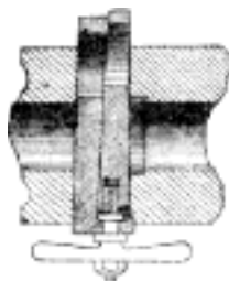
Č. 1090. Závěr dvojtypým klínem dle Kreinera.
