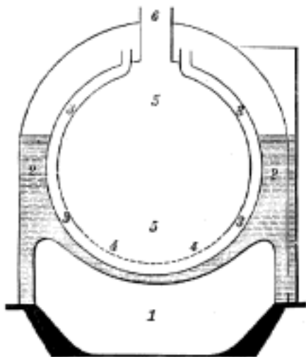
Č. 1118. Thursfieldův desinfekční přístroj v průřezu. 1. topeniště, 2. vodní plášť, 3. pární roury, 4. otvory, jimiž pára vniká do prostoru desinfekční, 5. prostora desinfekční, 6. odvodná roura pro páru.
