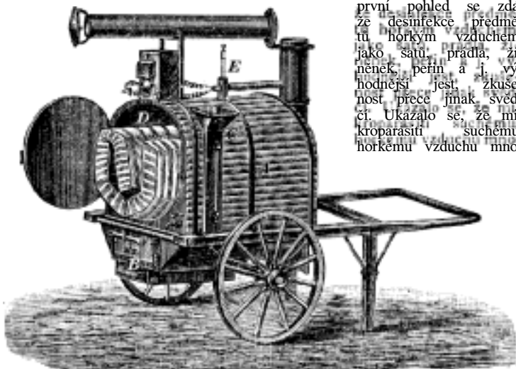
Č. 1119. Desinfekční přístroj Thursfieldův. A plášť kotlu, B topeniště, C otvor a roura, kterou se nalévá voda, D prostora desinfekční, E teploměr.
