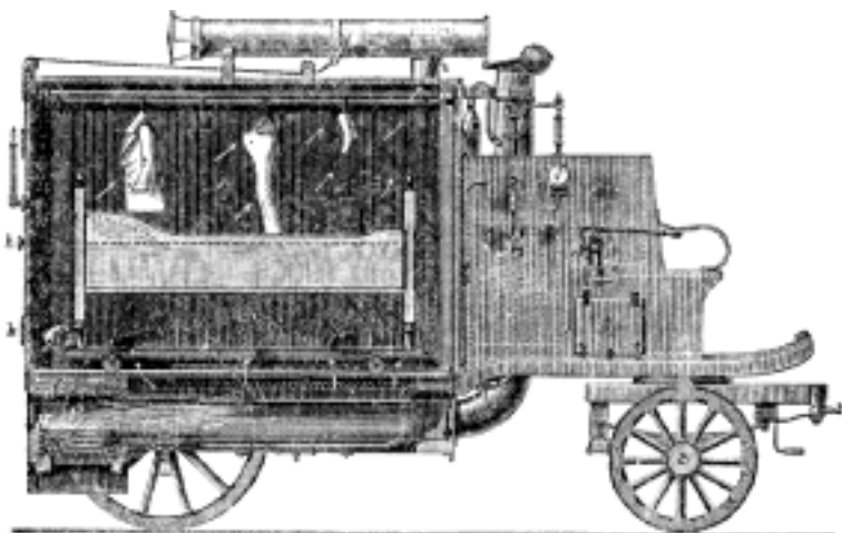
Č. 1120. Desinfekční přístroj Schäffer-Walckerův. F topeniště, H hadovité roury na svinování páry, t teploměr, h dveře ku prostoru desinfekční.
