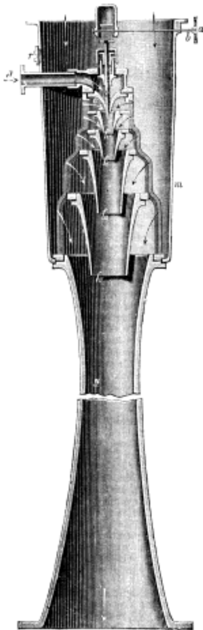
Č. 1176. Dmychadlo parotryskové (Körtingovo).
