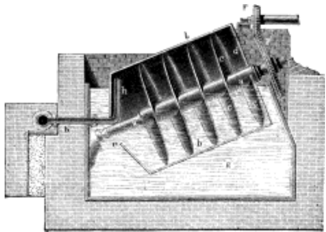
Č. 1174. Dmychadlo závitové (cagnardella).
