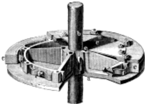
Č. 1171. Plátěné ucpání pístu dmychadel cylindrových.
