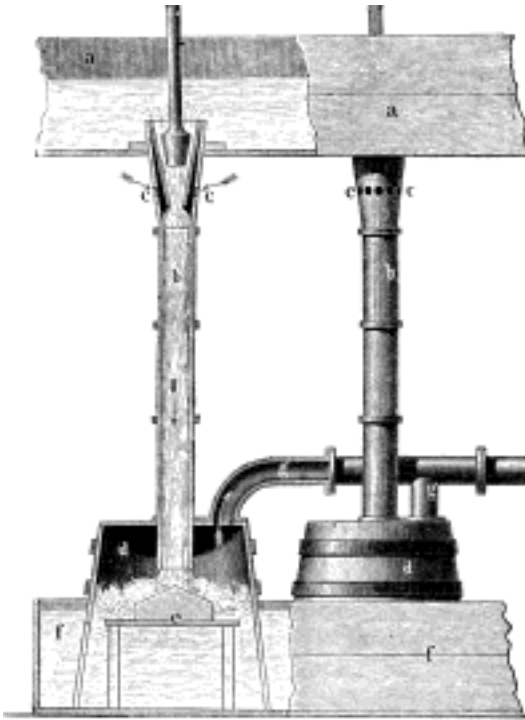
Č. 1173. Dmychadlo vodotrubné.
