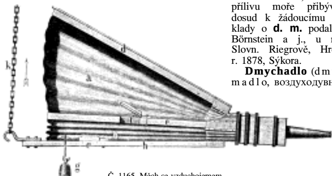
Č. 1165. Měch se vzduchojemem.
