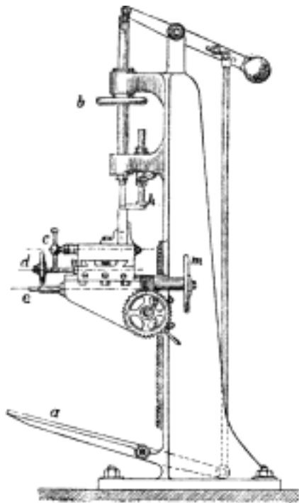
Č. 1160. Dlabací stroj.
