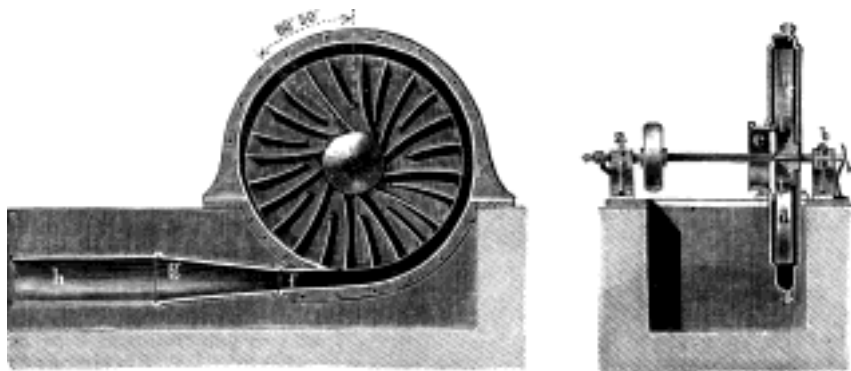
Č. 1175. Rittingerův větrník.
