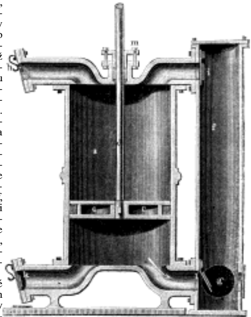
Č. 1169. Dmychadlo cylindrové čili válcové (stojmé).
