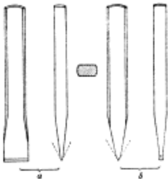
Č. 1161. Dláta na kovy.
