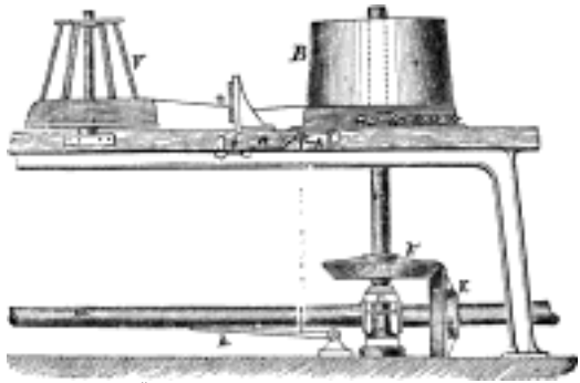
Č. 1220. Tažní lavice pro drát železný.
