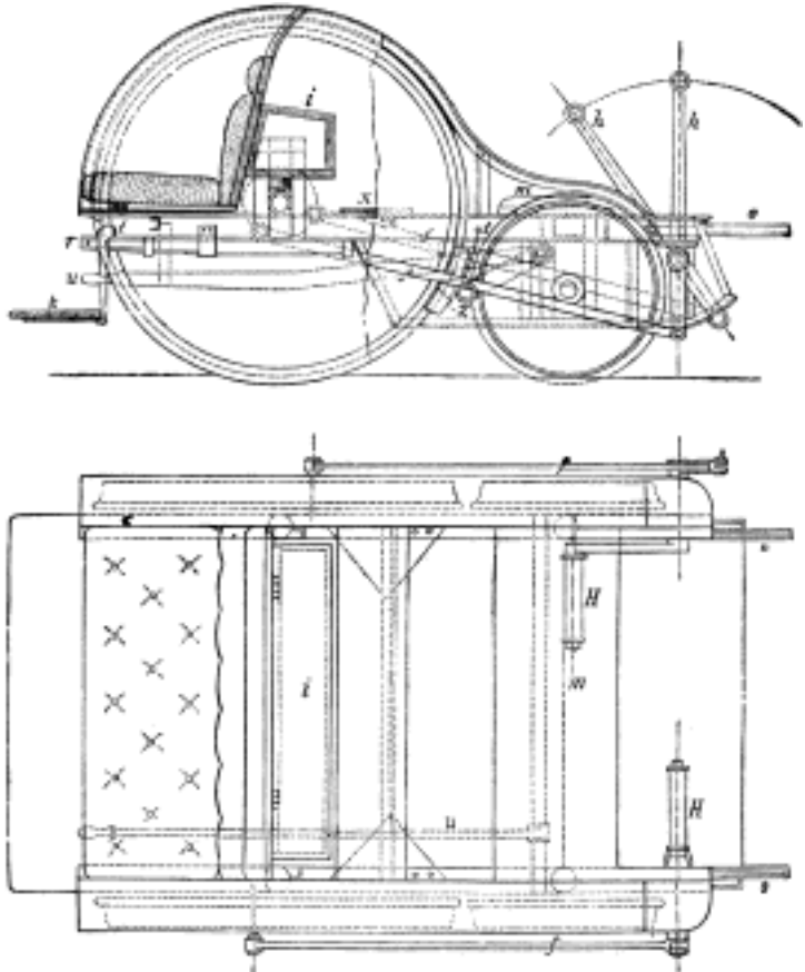
C. 1218. Leonhardiho draisina (1 : 30).
