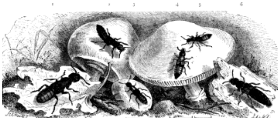
3 4 5 6 Č. 1212. Drabčící. 1. Svinonožec smrdutý ( Ocypus olens Müll.). - 2. Drabčík srstnatý ( Staphylinus pubescens De Geer.). - 3. Lejnomoil kovový ( Philonothus aeneus R.). - 4. Kráčivec červený ( Oxyporus rufus L.). - 5. Rudoštitník pobřežní ( Paederus riparius L.). - 6. Drabčík císařský ( Staphylinus caesareus Ced.). - Obr. 3., 4. a 5. slabě zvětš.
