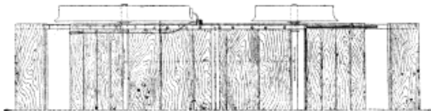
Č. 1217. Plankova draisina (1 : 30).
