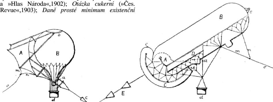
Č. 4942. Douglastův drak ballonový. Č. 4943. Parsevalův drak ballonový.
