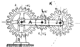
Č. 4939. Houldsworthův mechanismus.
