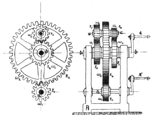
Č. 4938. Differenciální soukolí s cylindrickými ozubenými koly.
