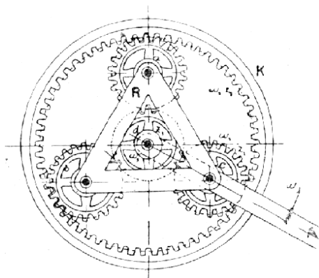
Č. 4940. Garrettův mechanismus.
