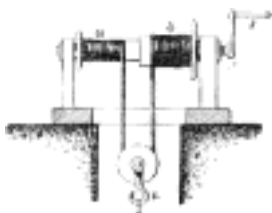
Č. 4937. Differenciální buben.
