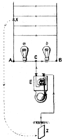
Č. 5021. Automatický přístroj k ohlašování poruch v izolaci.
