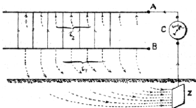
Č. 5020. Měření izolace elektrické sítě v chodu.
