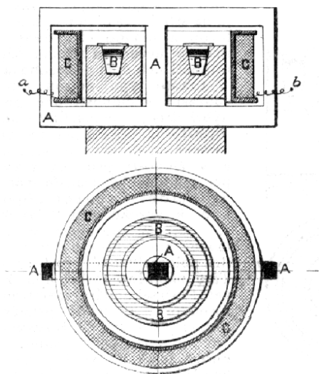
Č. 5002. Colbyho pec indukční.
