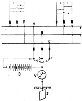
Č. 5019. Měření izolace elektrické sítě třívodičové.
