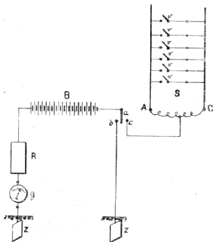
Č. 5017. Měření izolace elektr. sítě, když není v chodu.
