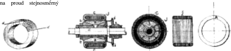
Č. 5008. Prstenový induktor. Č. 5009. Detailní uspořádání prstenového induktoru válcového.
