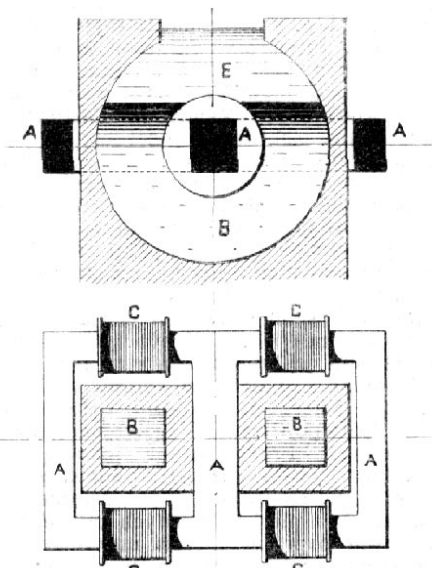
Č. 5006. Wallinova pec.
