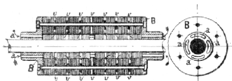
Č. 5013. Detailní uspořádání induktoru bubnového.
