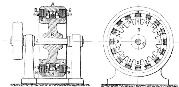
Č. 5015. Induktorový stroj.
