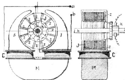
Č. 5007. Induktor stroje dynamoelektrického.
