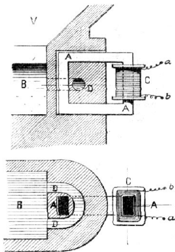
Č. 5005. Schneider-Creuzotova pec.
