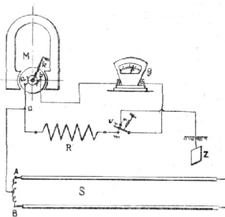
Č. 5018. Měření izolace sítě elektrické magnetoindukčním strojkem.
