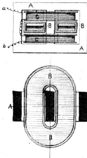
Č. 5001. Ferrantiho pec indukční.
