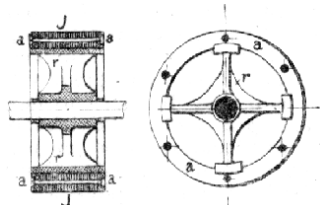
Č. 5010. Prstenový induktor válcový s rosetou.
