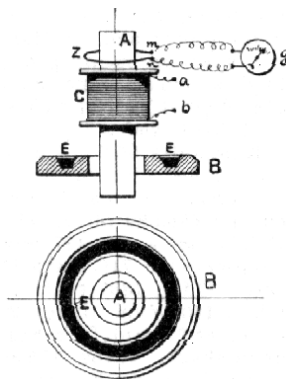
Č. 5000. Princip indukční peci.
