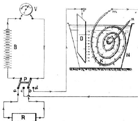
Č. 5016. Měření izolace kabelu před uložením do země.
