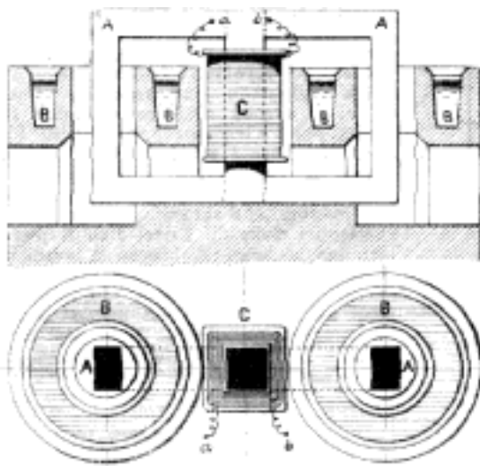
Č. 5004. Hiorthova pec.
