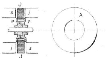
Č. 5011. Kotoučový induktor prstenový.
