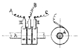
Č. 5037. Sběrací kroužky konvertoru.
