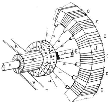
Č. 5031. Kolektorový stroj.
