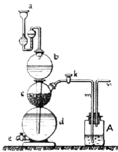
Č. 5028. Kippův přístroj.
