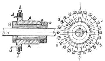
Č. 5032. Detailní uspořádání kolektoru.
