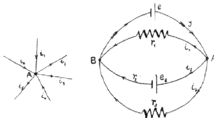
Č. 5029. První zákon Kirchhoffův. Č. 5030. Druhý zákon Kirchhoffův.
