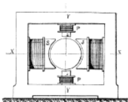
Č. 5033. Kompensační póly.
