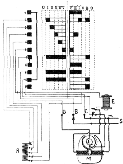
Č. 5035. Vnitřní zařízení kontroloru.
