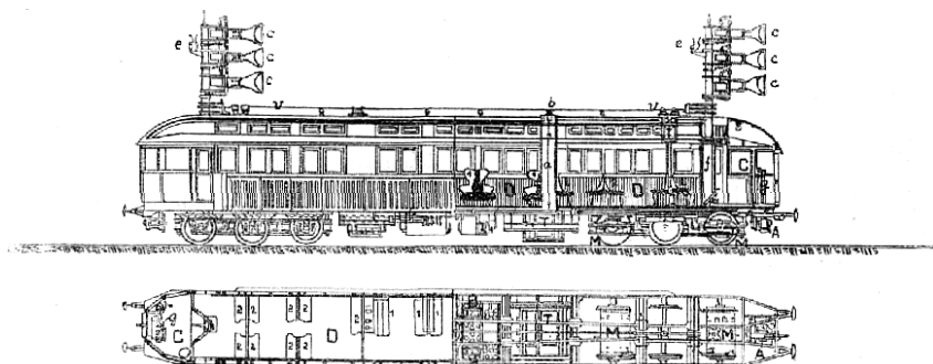
Č. 5049. Elektrický motorový vůz rychlikový.
