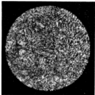
Č. 5046. Zakalená ocel nástrojová. Martensit.
