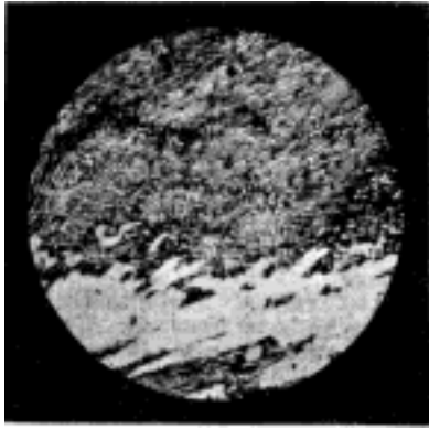
Č. 5045. Ocel s více než 0,95 % uhlíku. (Bílá plocha volný cementit, ostatní páskový perlit.)
