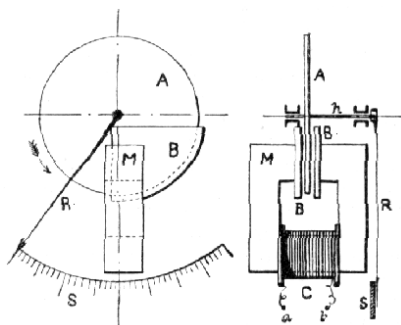
Č. 5041. Elektroindukční princip.
