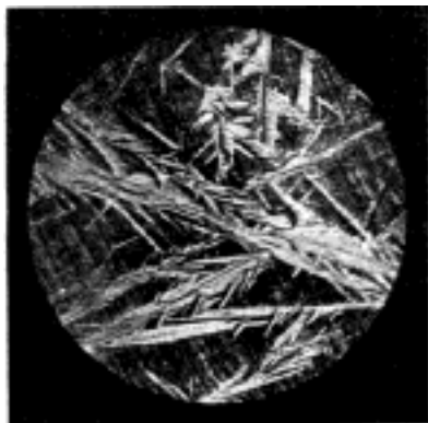
Č. 5047. Zakalená ocel nástrojová s 1,5% uhlíku. (Bílé je martensit, tmavé austenit.)
