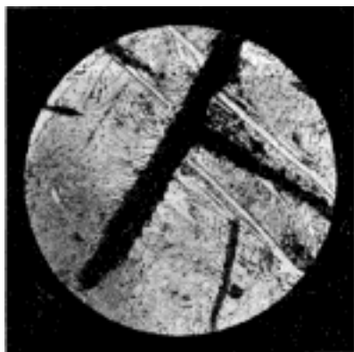
Č. 5048. Šedé železo surové. (Černé žíly grafit, světlé cementit, ostatek páskový perlit.)
