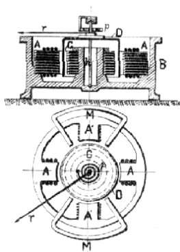
Č. 5042. Ferrarisův princip.
