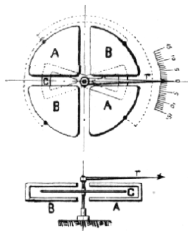
Č. 5040. Princip elektrostatický.
