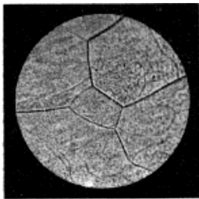
Č. 5043. Ferrit. (Charakterisují jej polygonální obrazy vzniklé leštěním a leptáním.)
