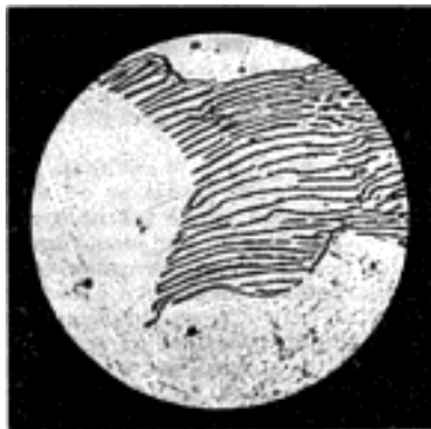
Č. 5044. Ocel s méně než 0,95% uhlíku. (Bílá plocha ferrit, ostatní páskový perlit.)
