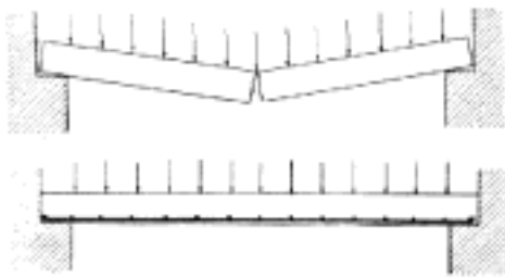
Č. 5056. a 5057. Armatura desky jakožto nosníku prostého.
