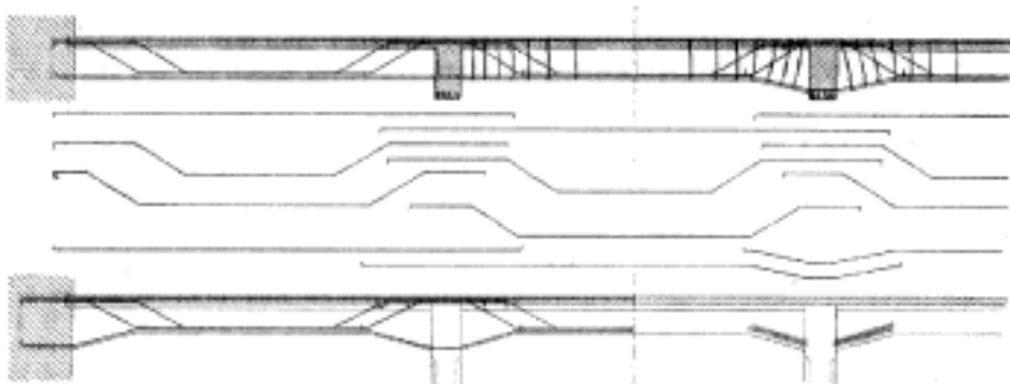
Č. 5062. Armatura desky ve spojení s trémem.
