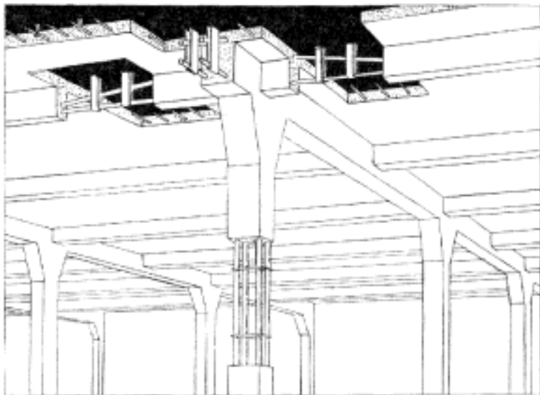
Č. 5066. Soustava Hennebiqueova.
