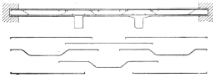
Č. 5060. Výztuhy desky jakožto nosníku spojitého.
