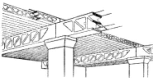
Č. 5067. Soustava Visintiniho.
