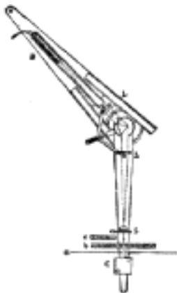
Č. 622. Spectro-bolometr (s hranolem ze soli kamenné).
