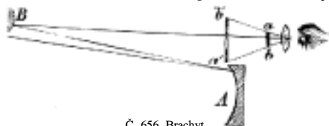
Č. 656. Brachyt.
