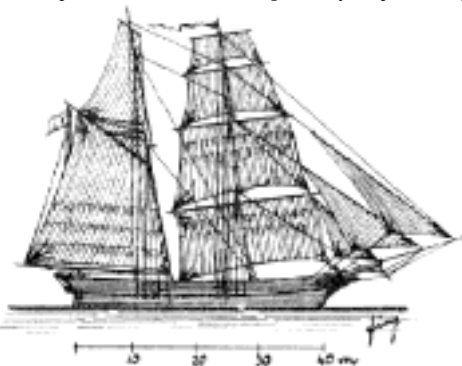
Č. 681. Brigschooner.
