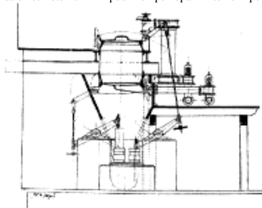
Č. 696. Bromovského diffusor.
