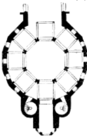
Č. 770. Půdorys kaple cisařské v hl. chrámě cášském.
