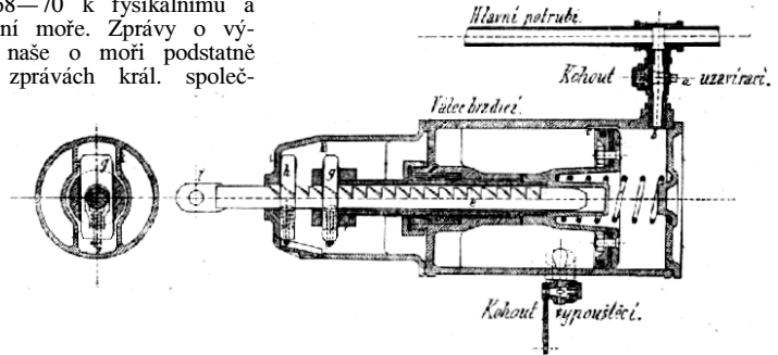
Č. 797. Carpenterova brzda.
