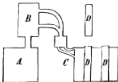
Č. 799. Schema Carréova stroje.
