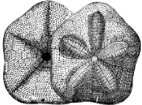
Č. 866. Clypeastridae: Clypeaster grandiflorus Bronn z útvaru třetihorního; zdola a shora.
