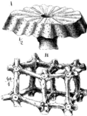
Č. 872. Coeloptychium decimum Gf. A) v pol velikosti, B) část kostry 40krát zvětš.
