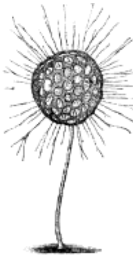
Č. 856. Clathrulina elegans Cienk., mřížinka stopkatá, zvětš.
