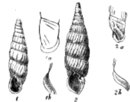
Č. 857. 1) Clausilia laminata Mont.; i a) spodní část' od zadku se 4 záhyby hltanovými; i b) závorca ( clausilium ); 2) Clausilia biplicata Mont.; 2 a) spodní část' od zadku se 2 záhyby hltanovými a s příčkou srpovitou; 2 b) závorca. Zvětšeno.
