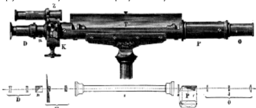
Č. 918. Cukroměr polostínový bratří Jos. a Jana Fričů v Praze.
