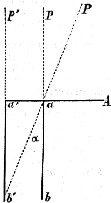
Č. 16. Aberrace světla.
