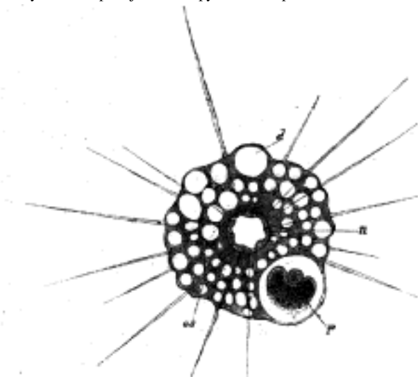
Č. 53. Actinophrys sol Ehrbg. n) jádro, d) stažená bublina, os) osní vlákénko panožky, p) potrava.
