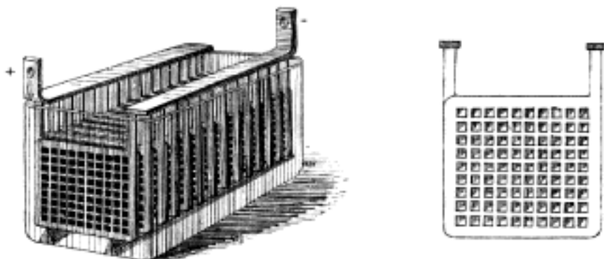
Č. 138. Elektrický akumulátor Faure-Sellon-Volckmarův.
