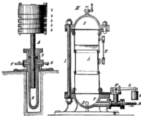
Č. 135. Č. 136. Akkumulátory hydraulické.
