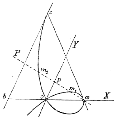
Č. 4014. Strofoida.
