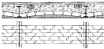
Č. 4028. Strop podle Hönela.
