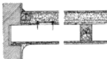
Č. 4017. Strop trámový obyčejný.
