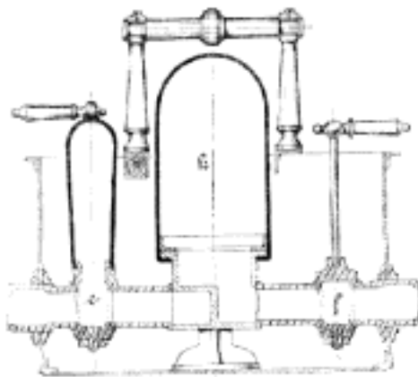
Č. 4012. Normální čtyřkolová vozová stříkačka. Č. 4013. Detaily normální čtyřkolové vrtové stříkačky.
