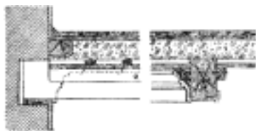
Č. 4019. Strop vídeňský.
