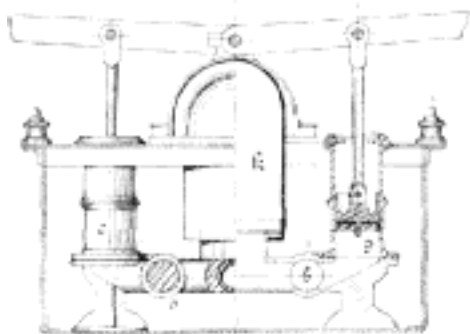
Č. 4012. Normální čtyřkolová vozová stříkačka. Č. 4013. Detaily normální čtyřkolové vrtové stříkačky.
