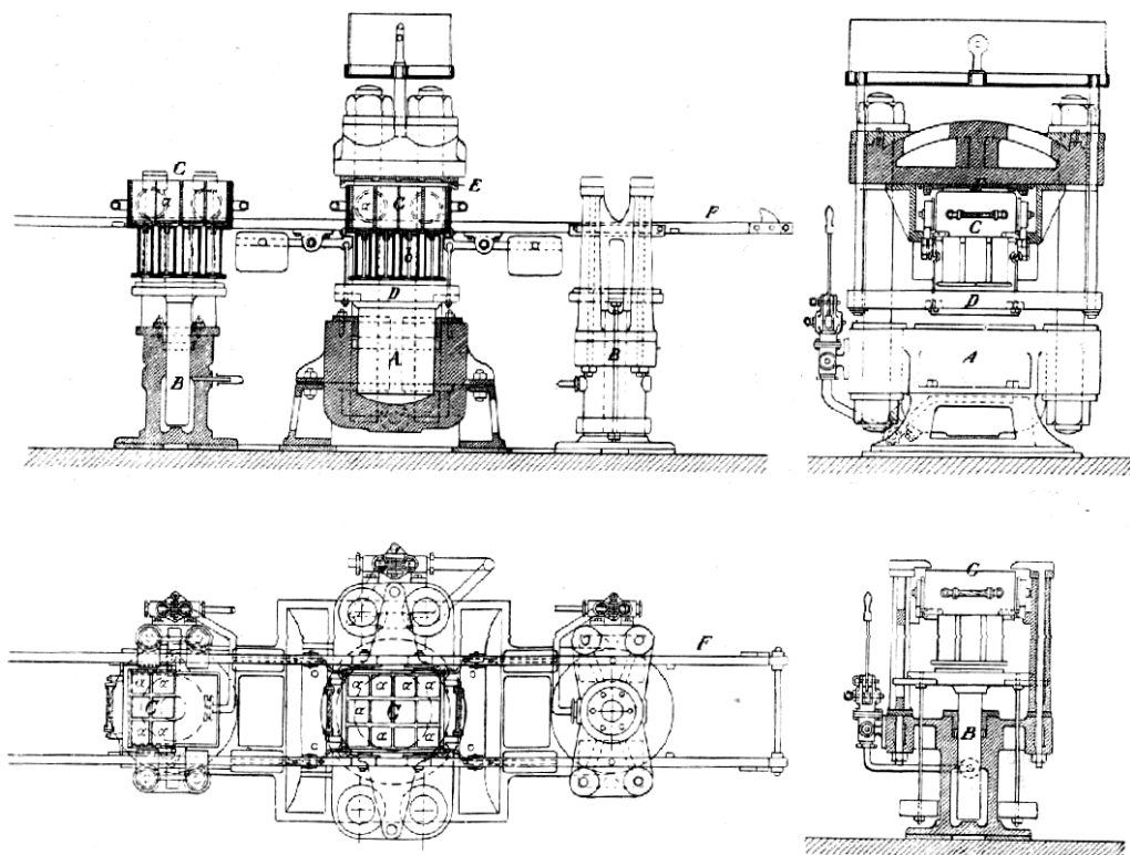
Č. 4049. Müllerův lis na kostky solné.
