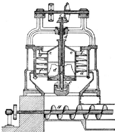
Č. 4056. Feskova diferenciální centrifuga.
