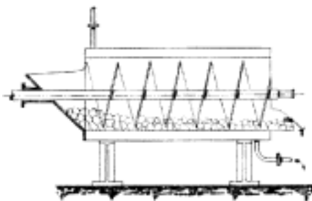
Č. 4064. Sušící buben nehybný.
