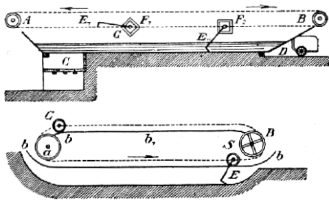
Č. 4055. Mechanické vytahování soli z pánve.
