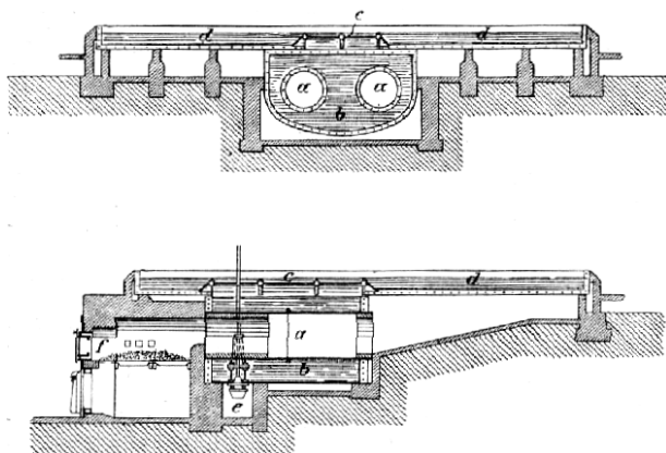
Č. 4054. Pánve systému Flaschendragerova.
