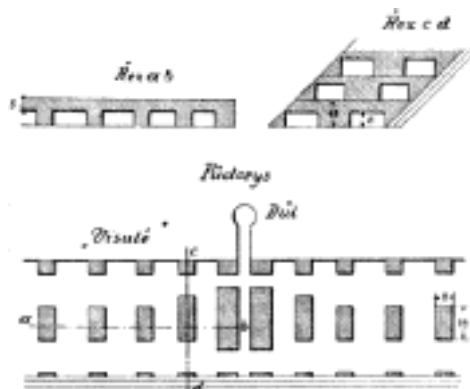
Č. 4040. Způsob dobývání soli.
