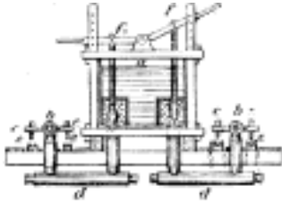
Č. 4043. Zařízení k uzavření přítoku rapy v gradovně.
