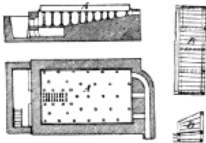
Č. 4046. Zařízení pánvi pro výrobu hurmanů.
