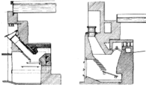
Č. 4052. Topení poloplynné k pánvi.
