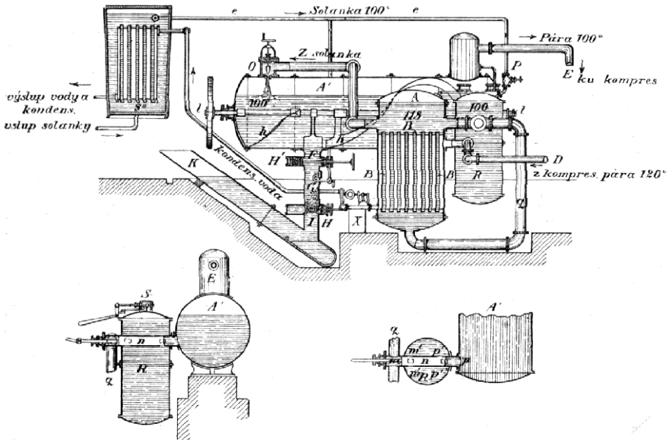
Č. 4057. Piccard-Weibelův odpařovací apparát.
