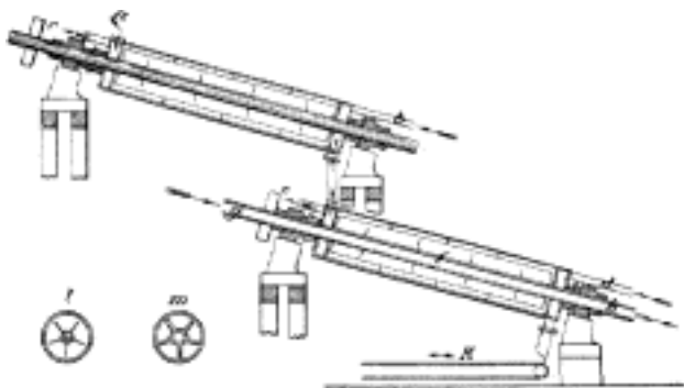
Č. 4048. Mechanické sušení soli.
