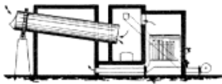
Č. 4063. Sušárna bubnová s kaloriferem a vnějším vytápěním pláště bubnového.
