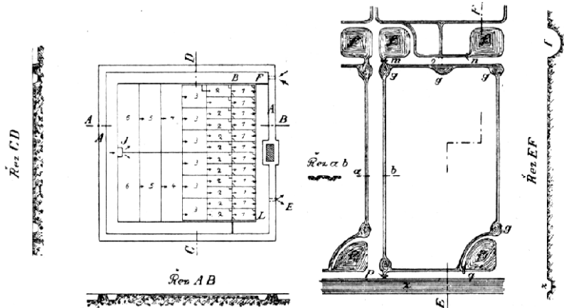
Č. 4045. Zařízení mořských salinek rakouských.
