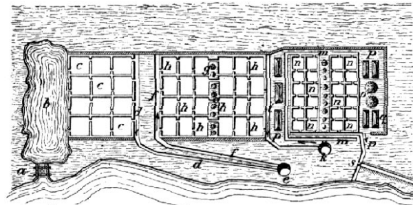
Č. 4044. Zařízení mořské salinky.
