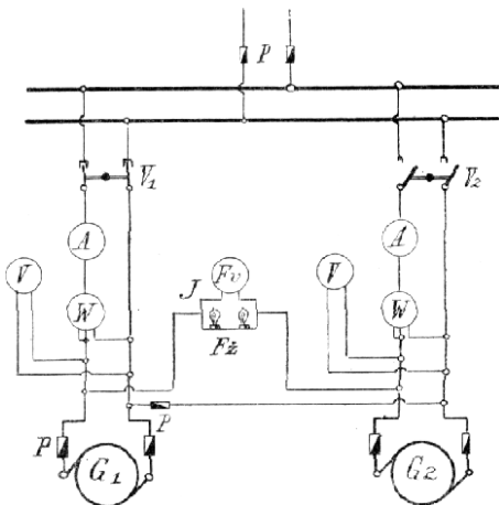
Č. 4079. Paralelní zapínání dynamoelektr. strojů jednofázových.
