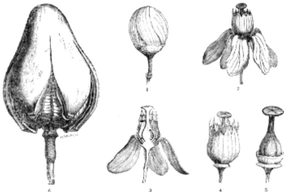
Č. 4077. Swietenia. 1. Květní pupen. 2. Květ. 3. Téžoz průřez podélný. 4. Pohár tyčinkový. 5. Semeník se žlaz. terčem. 6. Plod podvojnými chloupky zdola se pukající.
