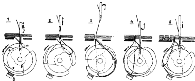
Č. 4091. Tvoření stehu kruhovým člunkem při strojích Wheeler-Wilsonových.
