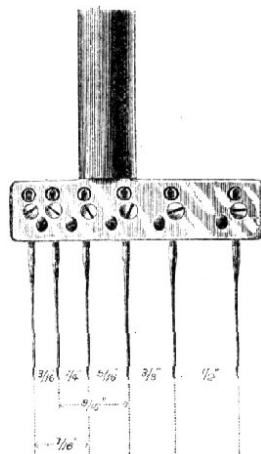
Č. 4085. Zakončení jehliště šicího stroje několikajehlového.
