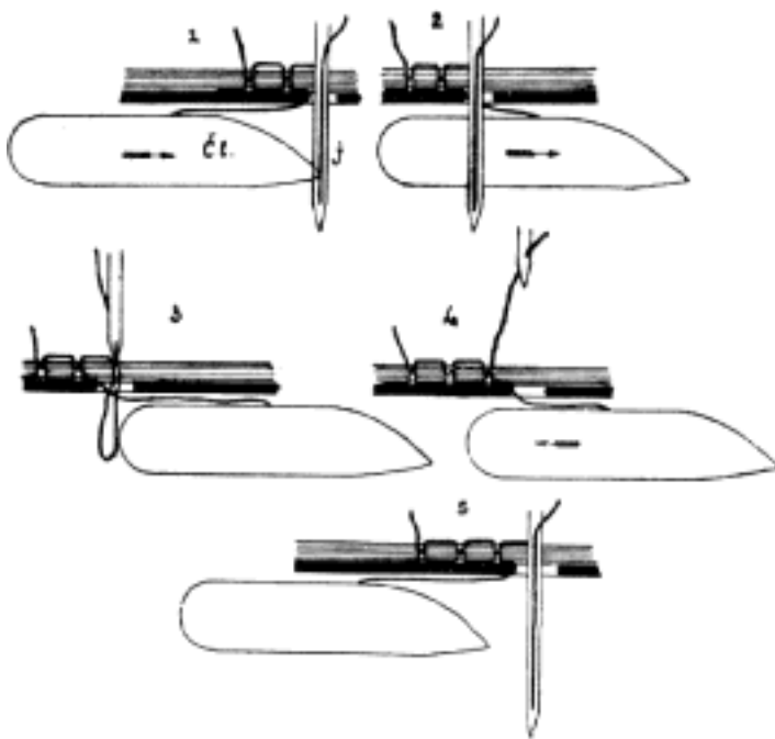
Č. 4090. Tvoření stehu dvojštepového pomocí člunku podélného.
