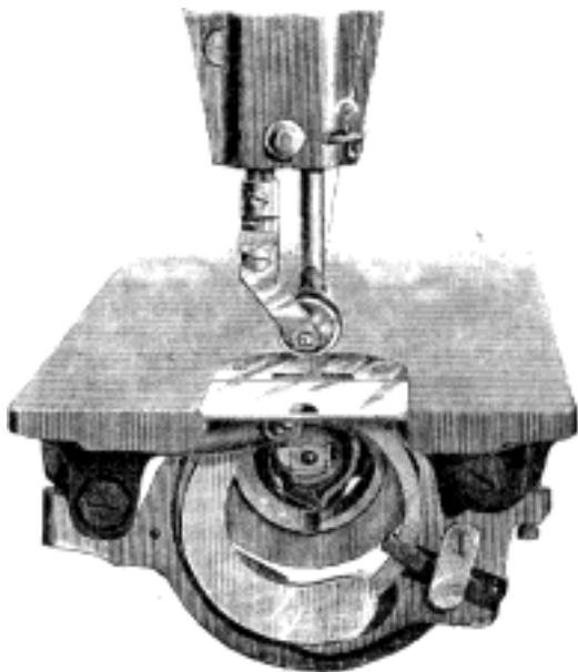
Č. 4103. Šicí ústrojí rychloběžného Singerova stroje s kolovým posouvačem, kolečkovou tlakovou nožkou s ústrojím »Central Bobbin«.
