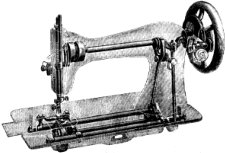
Č. 4100. Vnitřní ústrojí Singerova šicího stroje »Central Bobbin F«.
