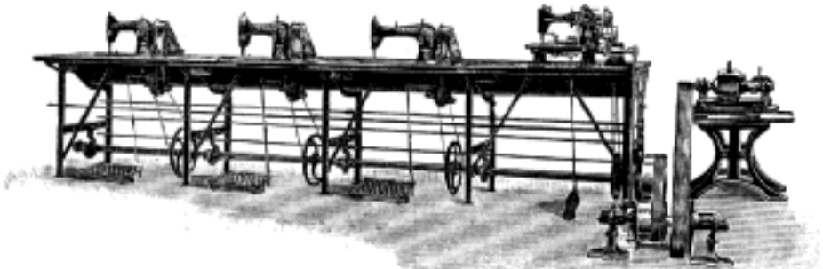
Č. 4101. Jednořadový pohon Singerových šicích strojů v upevněných na společném stole se žlabem.
