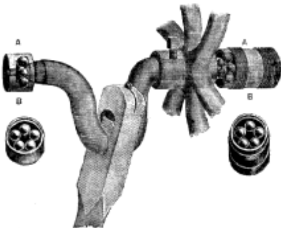
Č. 4099. Hřídelová klika Singerových šicích strojů s kuličkovými ložisky.
