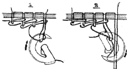
Č. 4095. Tvoření stehu dvojitěřetězového při stroji Grover-Backerově.
