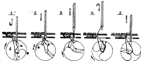
Č. 4093. Tvoření stehu řetězového při strojích Wilcox-Gibbsových.
