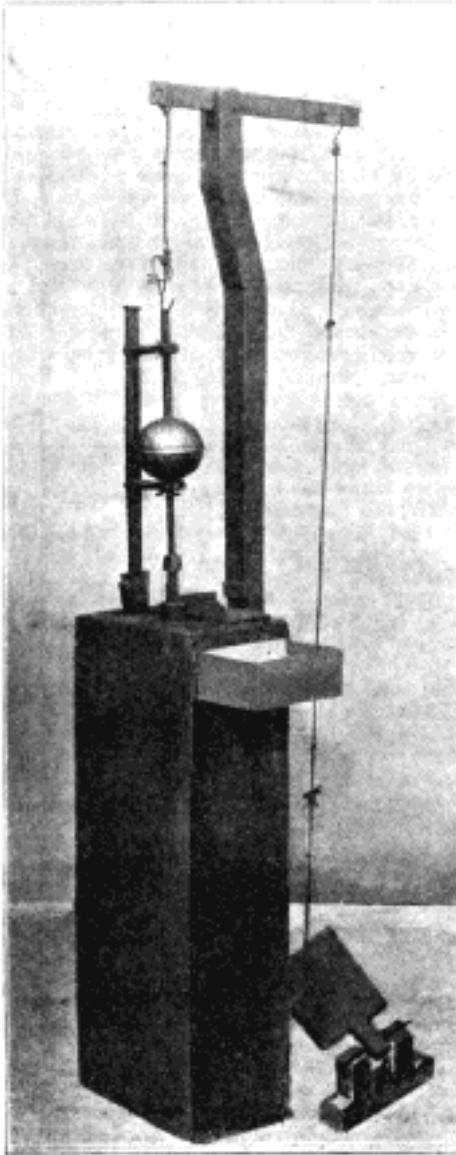
Č. 4118. Stroj přitloukací.
