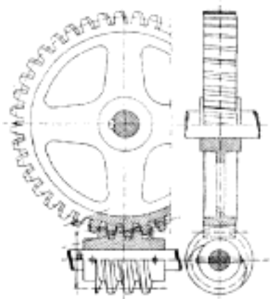
Č. 4134. Šroubové kolo.
