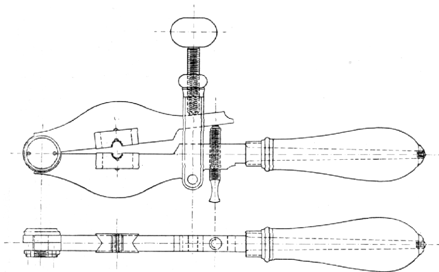
Č. 4128. Závitnice nůžková.
