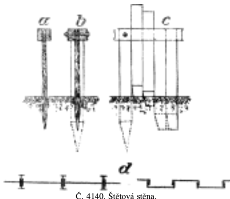
Č. 4140. Štětová stěna.
