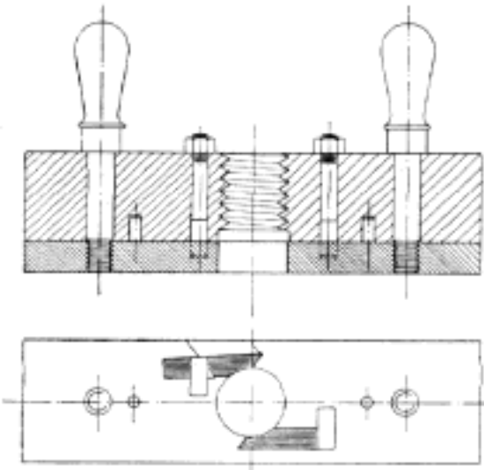
Č. 4131. Závitnice na řezání šroubů dřevěných.
