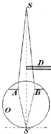
Č. 4163. Talbotovy proužky.
