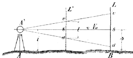
Č. 4160. Měření nitkovým dalekoměrem.
