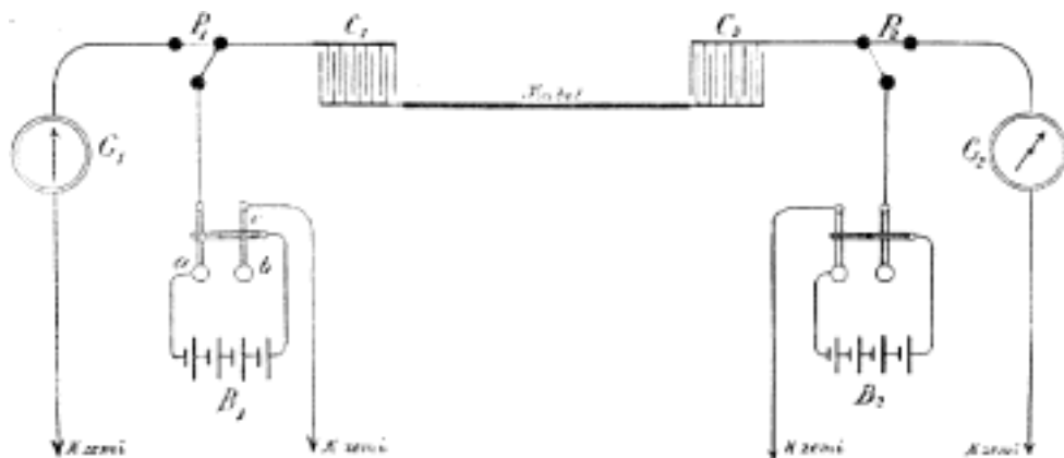
Č. 4213. Spojení při telegrafii kabelové.
