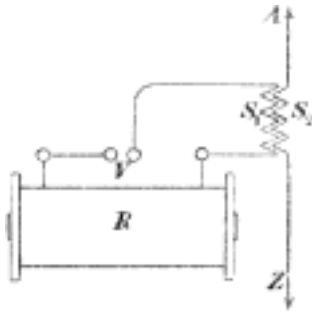
Č. 4217. Induktivní excitace.
