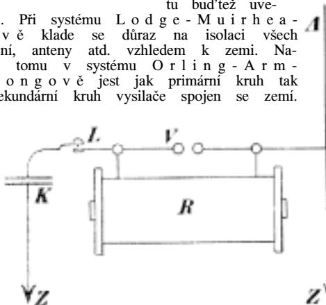
Č. 4219. Systém Slabý-Arco.
