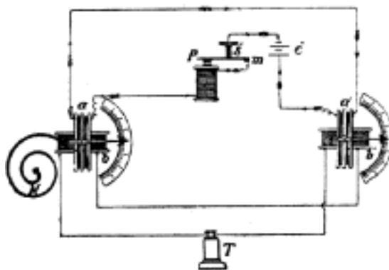
Č. 4246. Teleinduktor.
