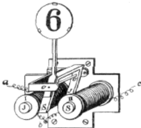
Č. 4227. Elektrický přístroj oznamovací.
