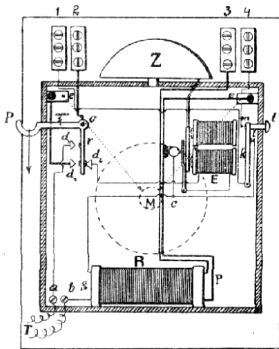
Č. 4199. Přístroj telefonní stanice domovní (vnitřní uspořádání).
