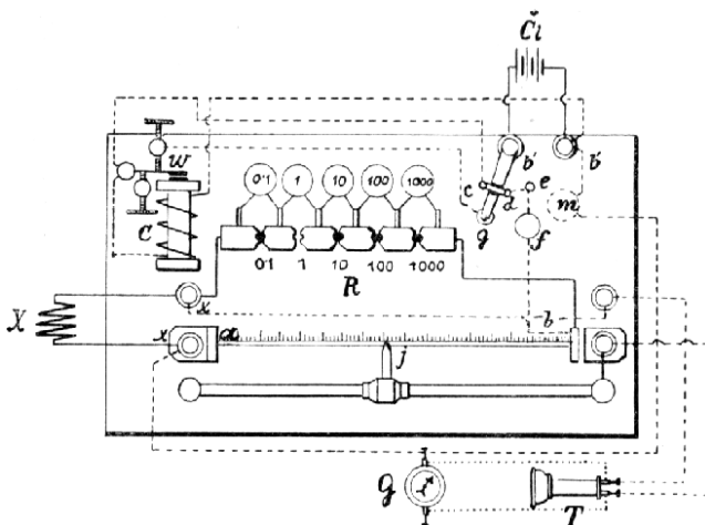
Č. 4195. Kohlrauschův můstek telefonní.
