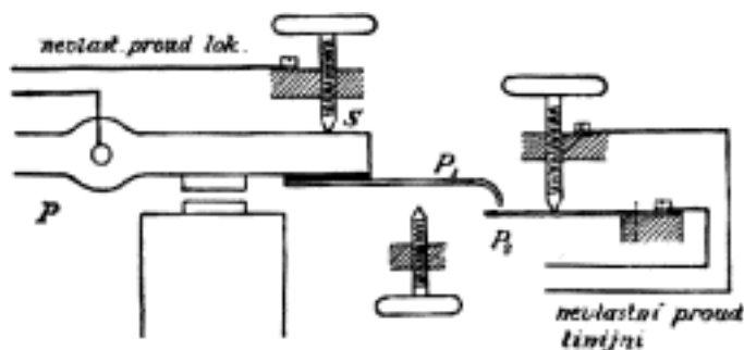
Č. 4243. Úprava Morseova přístroje pro úplnou translaci.
