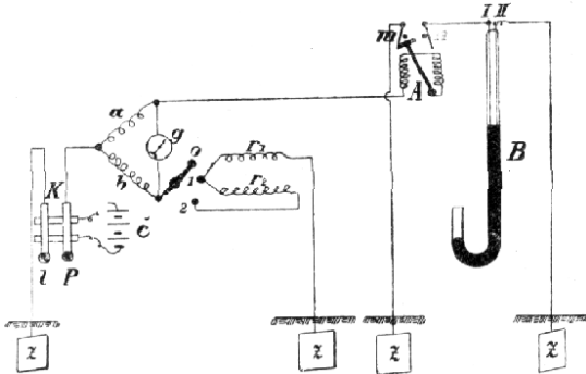
Č. 4187. Telebarometr.
