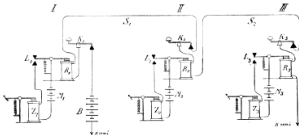
Č. 4208. Spojení proudem trvalým.
