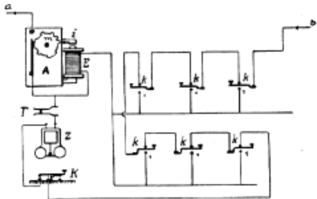
Č. 4236. Požární automat s poboční sítí oznamovací.
