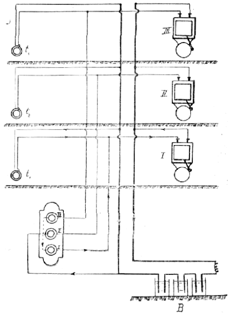
Č. 4230. Zařízení elektrického zvonku pro dům.
