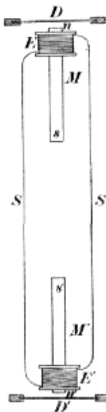
Č. 4189. Telefonické spojení dvou stanic.
