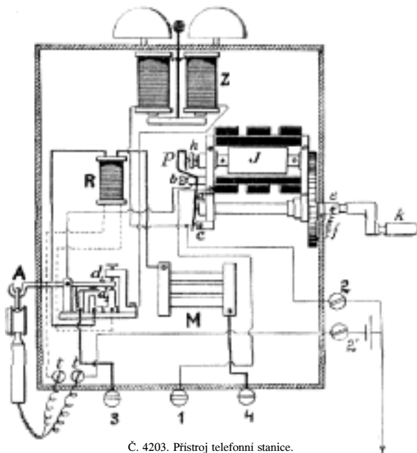
Č. 4203. Přístroj telefonní stanice.
