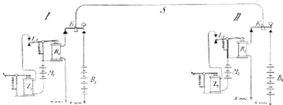
Č. 4209. Spojení proudem činným.
