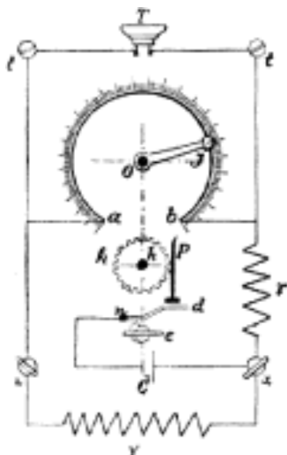
Č. 4196. Telefonní můstek Siemens-Halskeho.
