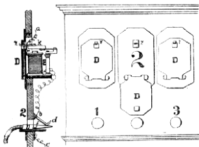
Č. 4204. Spojovací deska ústřední telefonní stanice.
