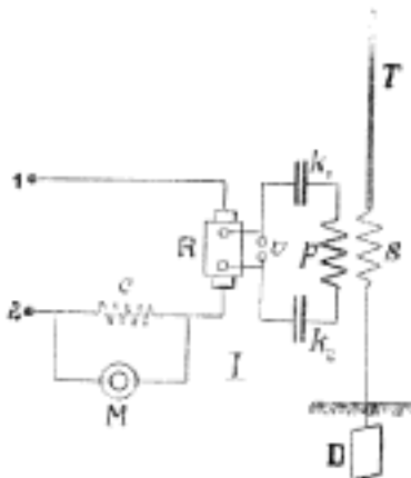
Č. 4194. Nussbaumerovo telefonování bez drátu.
