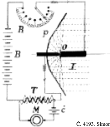
Č. 4193. Simonovo telefonování bez drátu.
