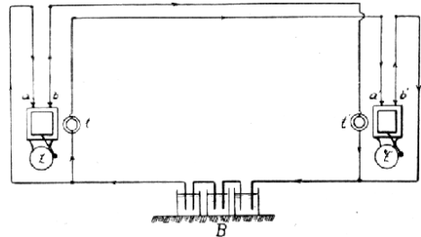
Č. 4231. Dvě stanice pro vzájemné signály s dvojitým vedením.
