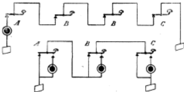
Č. 4237. Spojení telegrafní.
