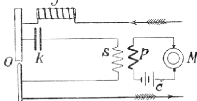
Č. 4192. Duddellovo uspořádání »mluvící lampy«.
