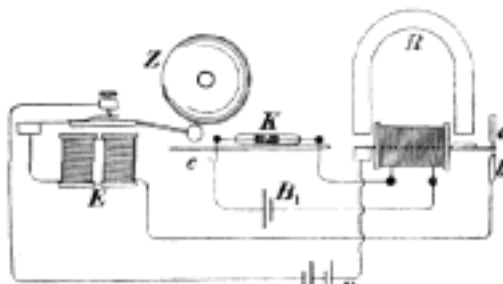
Č. 4215. Telegrafie bez drátu.
