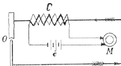
Č. 4191. Simonovo původní uspořádání »mluvící lampy«.
