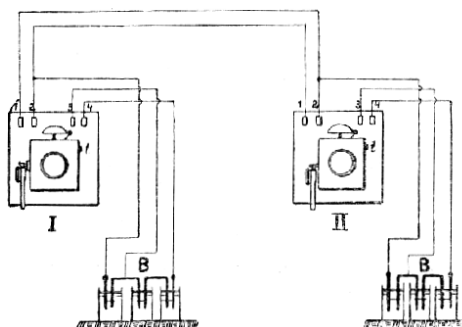
Č. 4201. Jednoduché spojení dvou telefonních stanic domovních.
