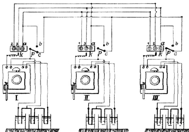
Č. 4202. Spojení několika telefonních stanic domovních pro důvěrný hovor.
