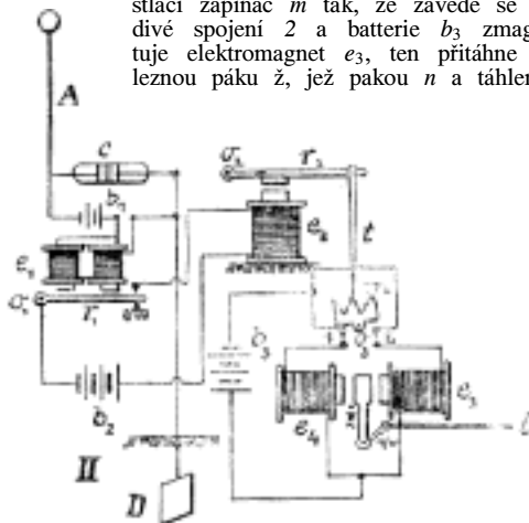
Č. 4221. Řízení torped telegrafií bez drátů.
