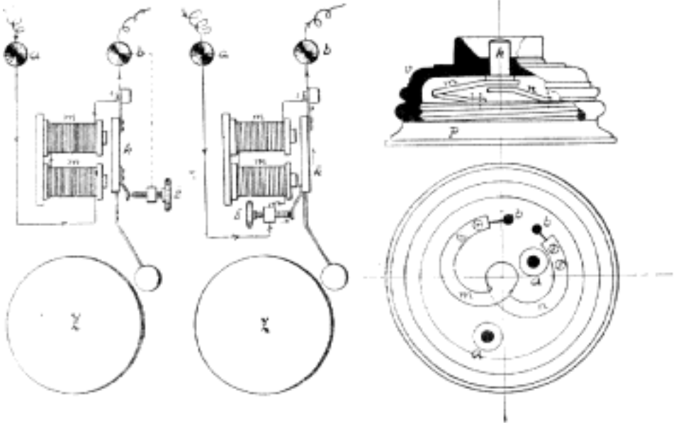
Č. 4221. Elektrický zvonek s jedním úderem. Č. 4222. Elektrický zvonek s paralelním spojením na krátko. Č. 4223. Obyčejné tlačítko nástěnné.
