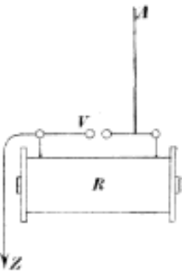
Č. 4216. Přímá excitace.
