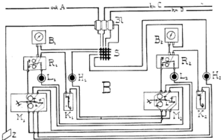
Č. 4242. Úplná translace.
