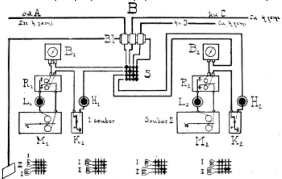
Č. 4240. Normální spojení přístrojů v odboční stanici.
