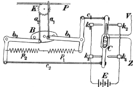
Č. 4212. Rychlotelegraf Wheatstoneův.
