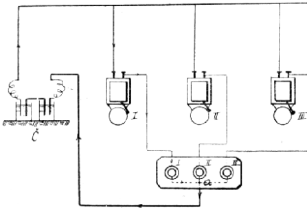
Č. 4229. Spojení několika elektrických zvonků k signalisování z jedné místnosti.
