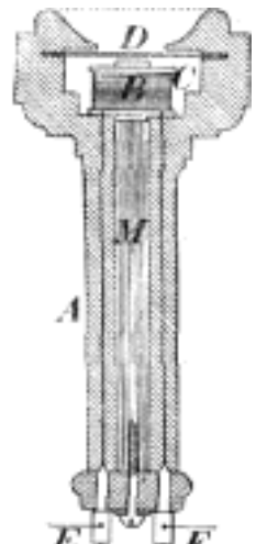
Č. 4188. Telefon Bellův.
