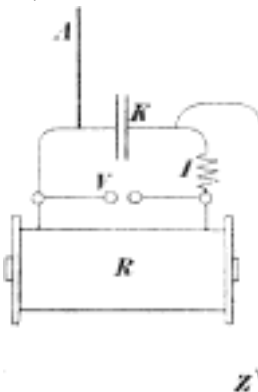
Č. 4218. Derivační excitace.
