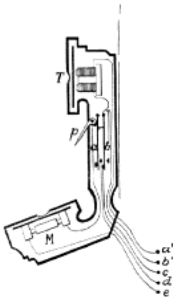
Č. 4200. Mikrotelefon čili telefon stolní.
