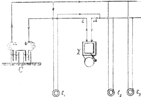
Č. 4228. Elektrický zvonek s několika tlačítky.
