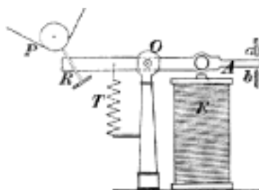
Č. 4207. Zapisovací přístroj telegrafický.
