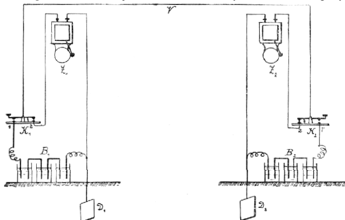
Č. 4232. Dvě stanice pro vzájemné signály s jedním vedením.
