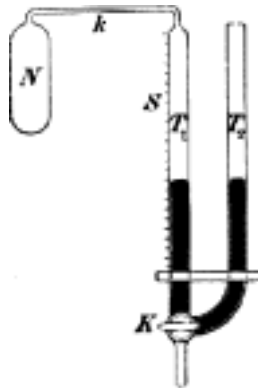
Č. 4254. Normální teploměr vodíkový na stálý tlak.
