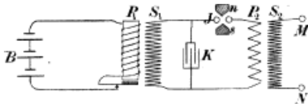
Č. 4267. Uspořádání pro teslovy proudy.
