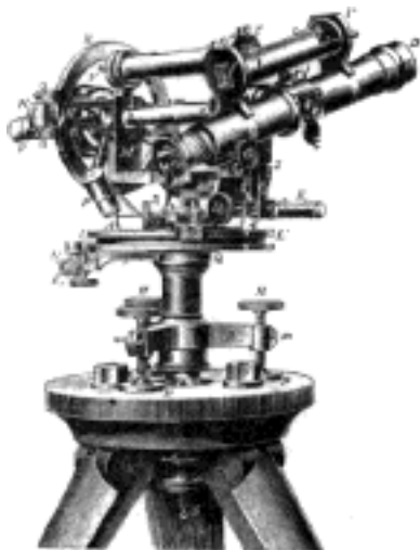
Č. 4290. Ertlův repetiční theodolit s excentrickým dalekohledem.
