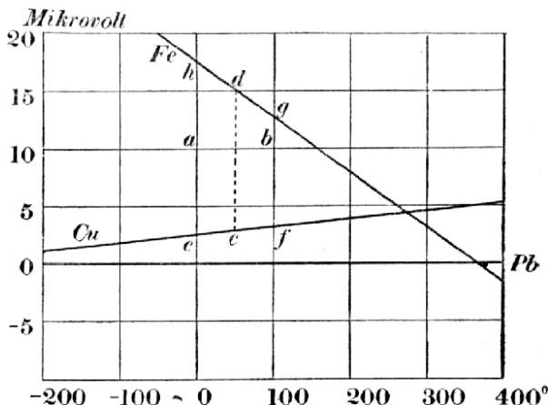
Č. 4295. Diagramm thermoelektrický.
