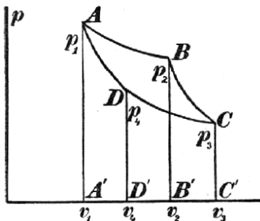
Č. 4292. Carnotův cyklus.
