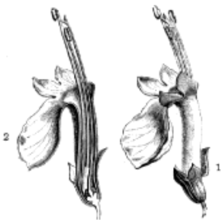
Č. 4285. Teucrium . 1. Květ celý, 2. v průřezu podélném.
