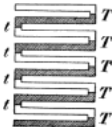
Č. 4294. Melloniho sloup thermoelektrický.
