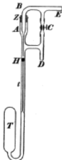
Č. 4300. Thermoregulátor.
