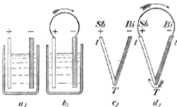
Č. 4293. Článek galvanický a thermoelektrický.
