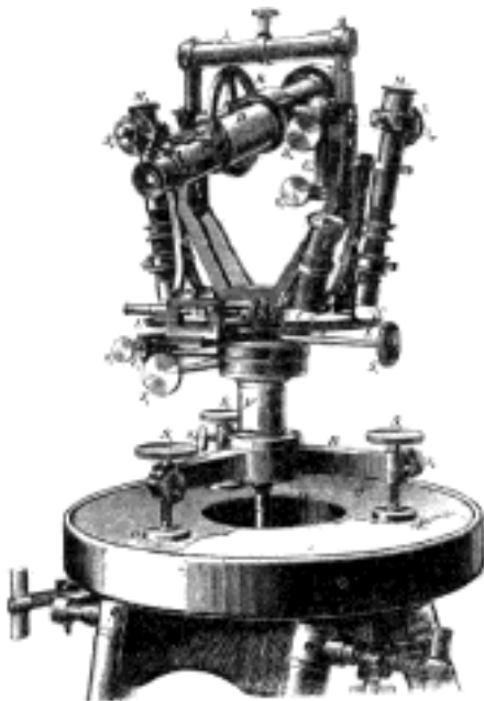
Č. 4291. Repetiční theodolit s nitkovými mikrometry.
