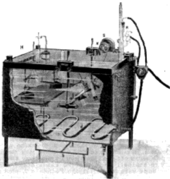
Č. 4299. Ostwaldův thermostat.
